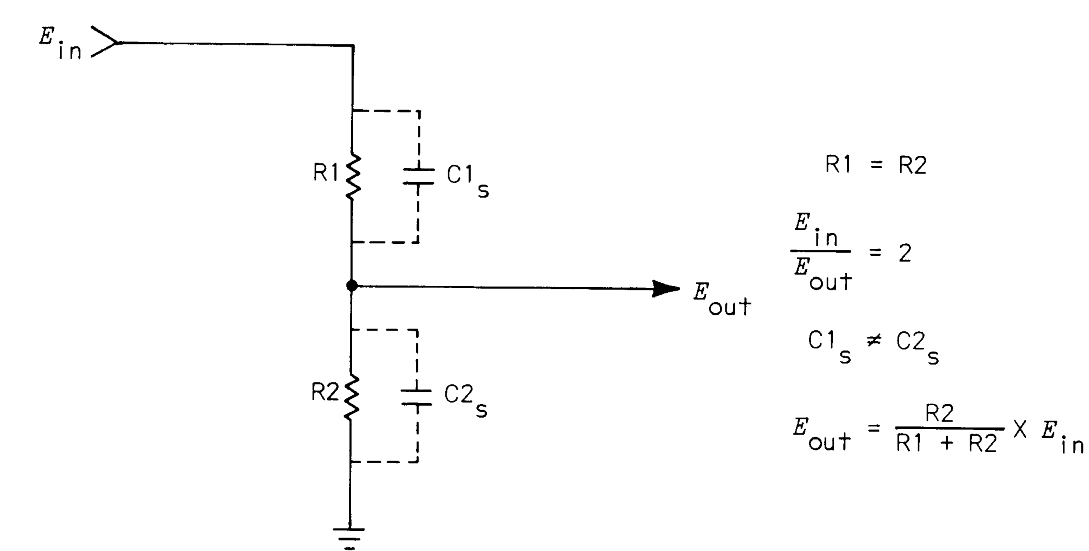
Fig. 1-4. Simple attenuator.
