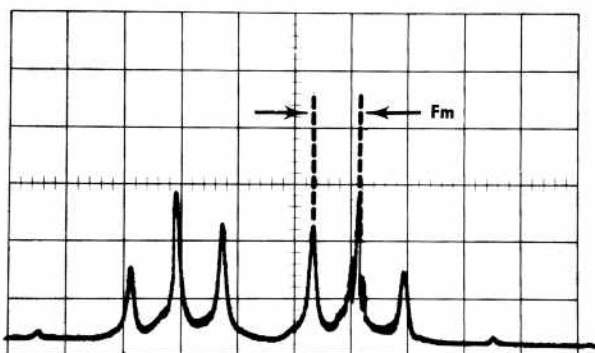
(D) Carrier at null.
