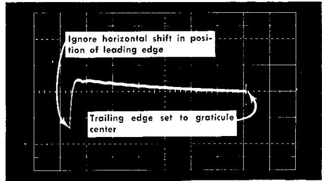
(D) Deflection factor 10 mV/div; sweep rate 1 \mu s/div
