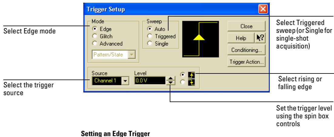
Setting an Edge Trigger
