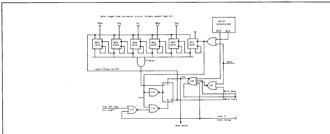
Figure 8—9—3. Exponent counter
