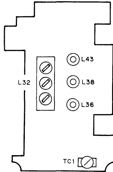
図 4 RF ユニット
