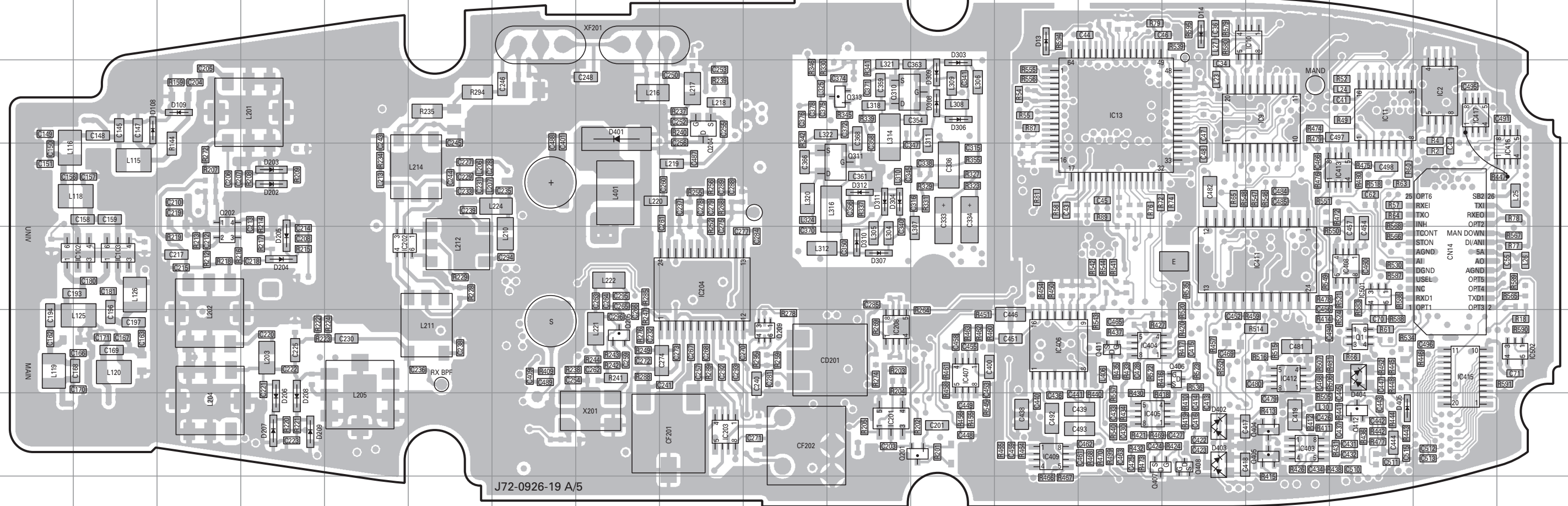
TX-RX UNIT (X57-6820-XX) (A/5) : TX-RX section -10 : K -11 : K2 -12 : K3 Component side view (J72-0926-19 A/5)
