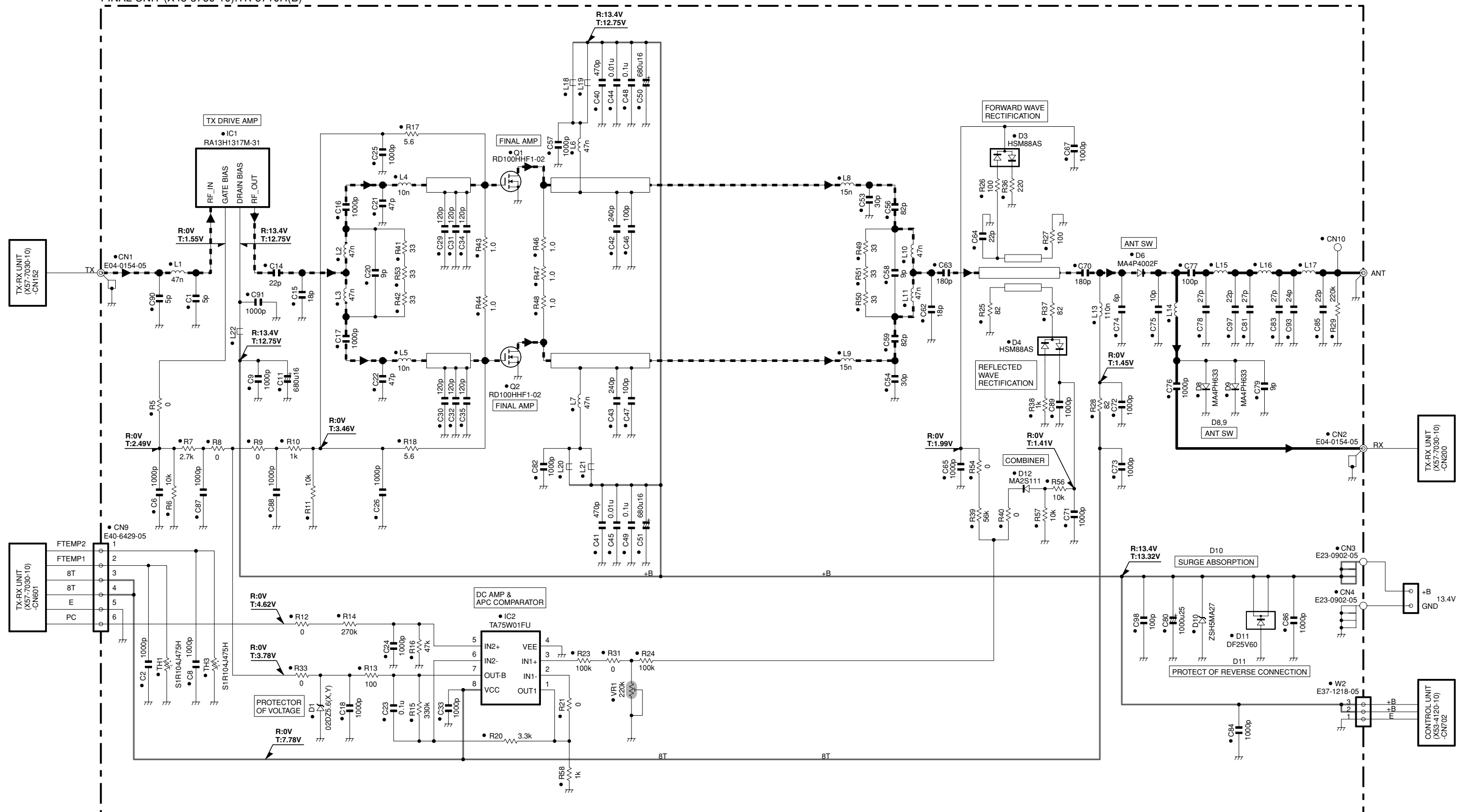
FINAL UNIT (X45-3760-10):TK-5710H(B)
