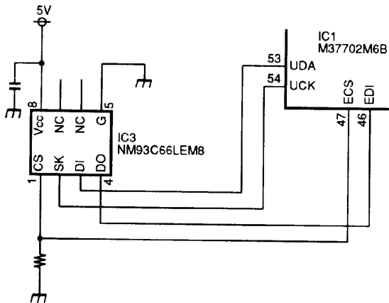
Fig. 19 EEPROM
