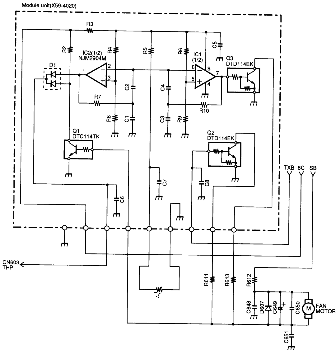
Fig. 11 Thermal protection
