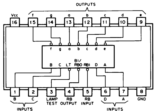
Fig. 8 SN74LS247N
