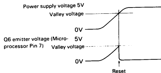
Fig. 11-A Reset timing
