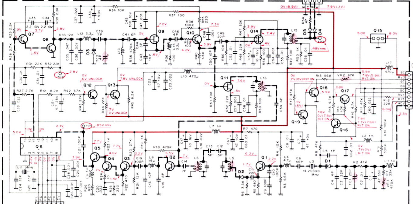
PLL UNIT (X50-1860-00)
