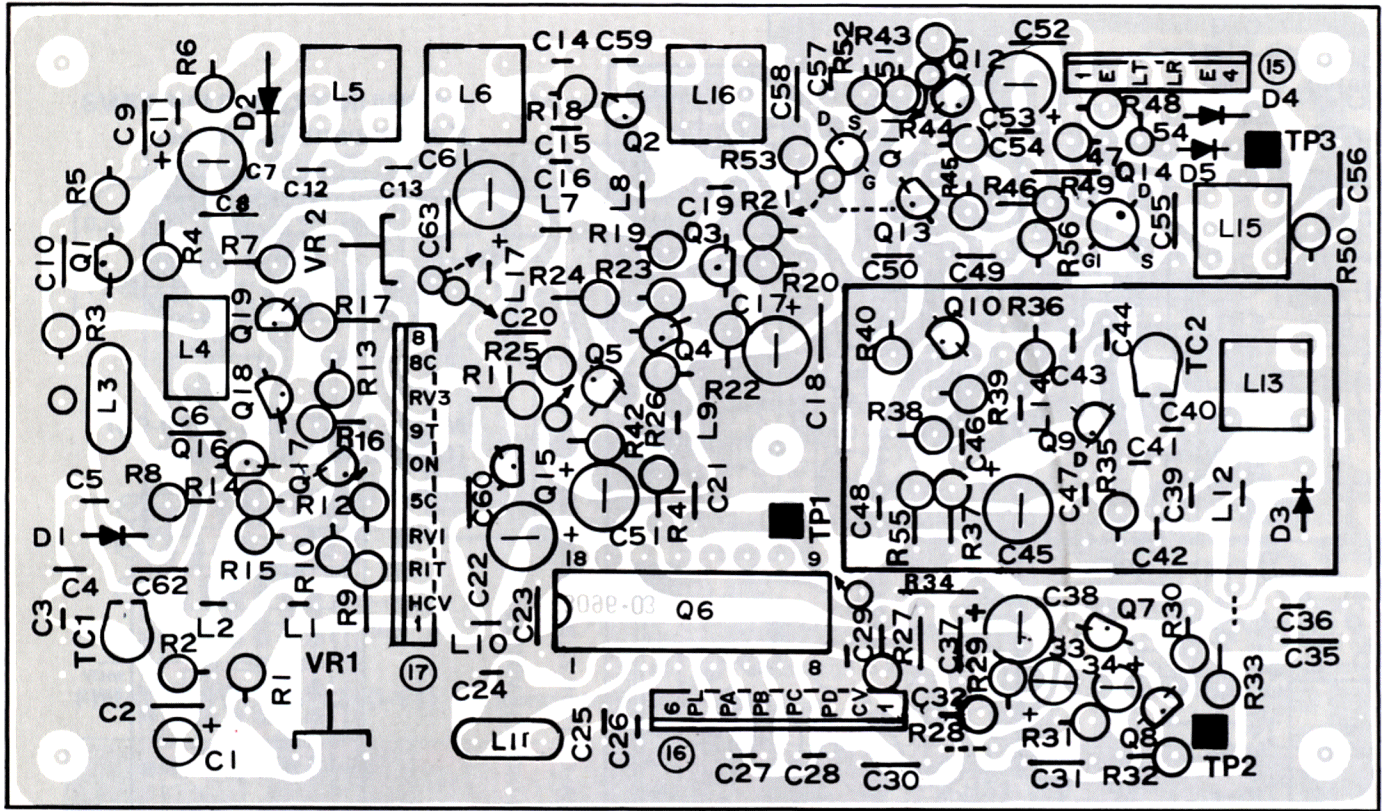
PLL UNIT (X50-1860-00)
