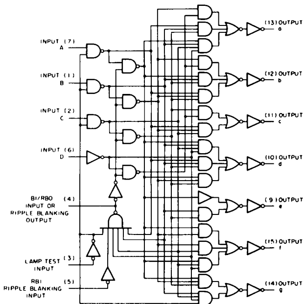
Fig. 7 SN74LS247N
