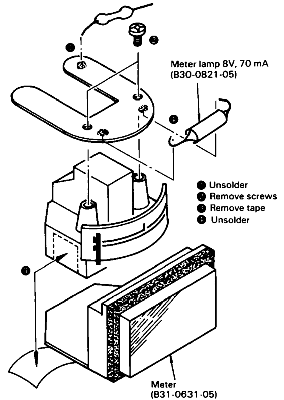
Fig. 17 Meter
