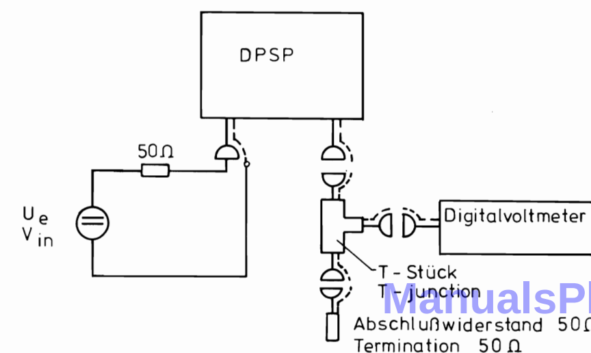
Bild 11 Prüfen der Dämpfungsglieder mit Gleichstrom Fig. 11 Checking the attenuator pads with DC
