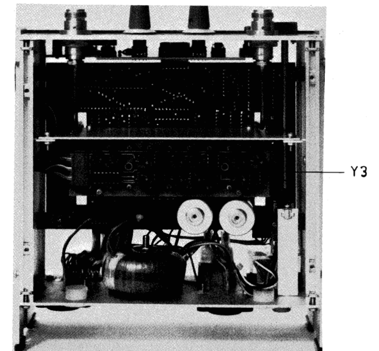
Bild 9 Innenansicht von unten Fig. 9 Interior view from below
