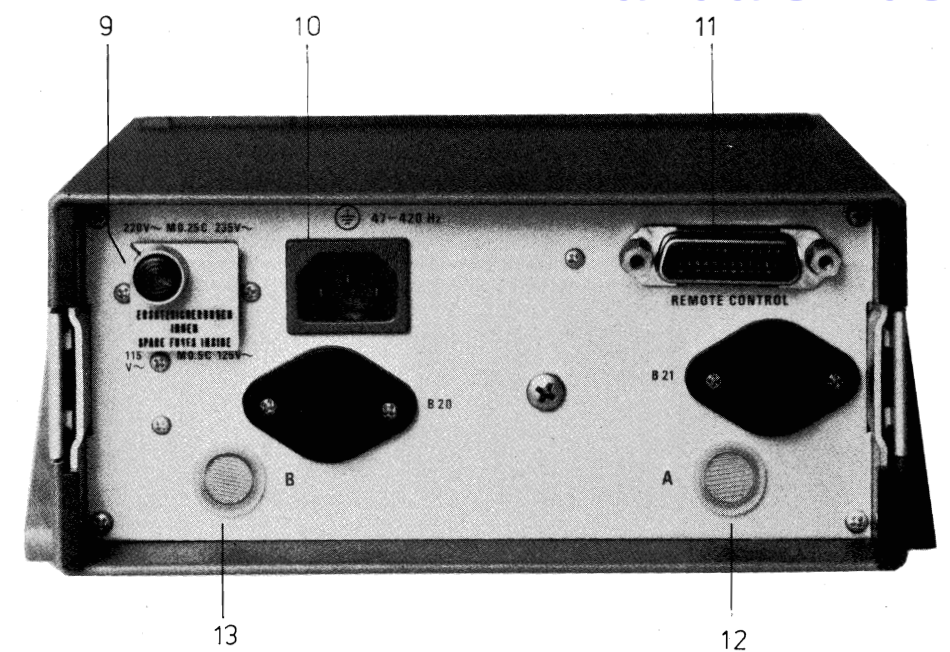
Bild 7 Rückansicht Fig. 7 Rear panel
