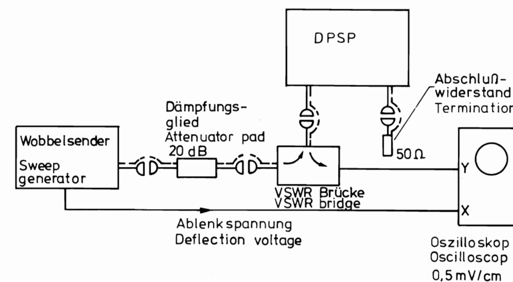
Bild 12 Prüfen des VSWR und der Schaltsicherheit Fig. 12 Checking the VSWR and the switching reliability
