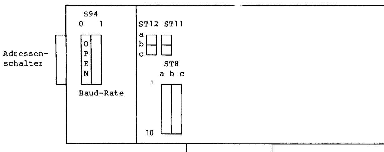
Bild 2.34 Lageplan der Kurzschluß-Stecker
