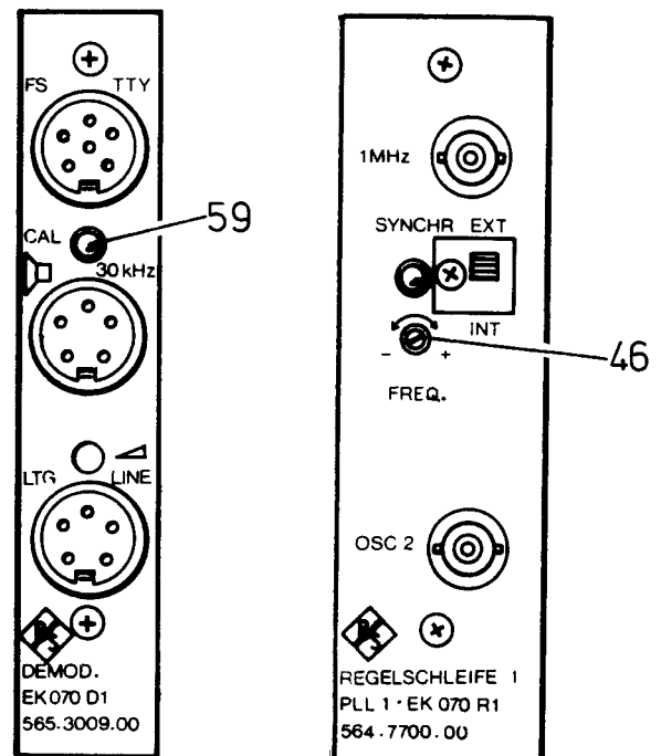
Bild 2.19 Frequenzkalibrierung
