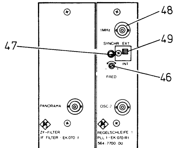
Bild 2.29 Normalfrequenzanschluß
