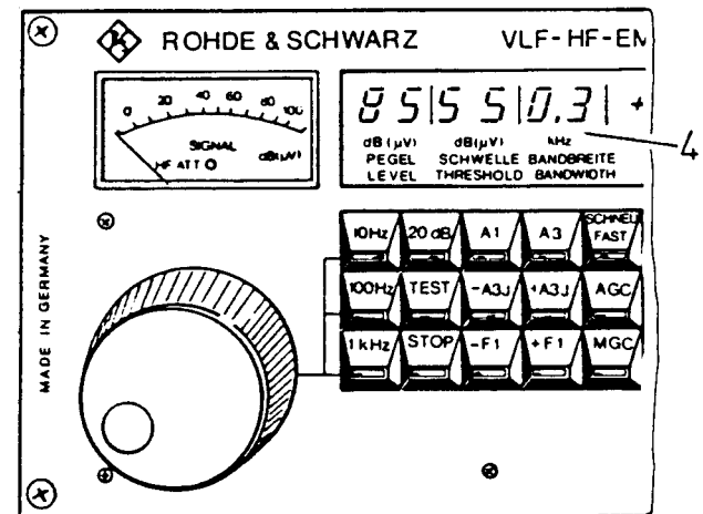
Bild 2.10 Bandbreitenanzeige
