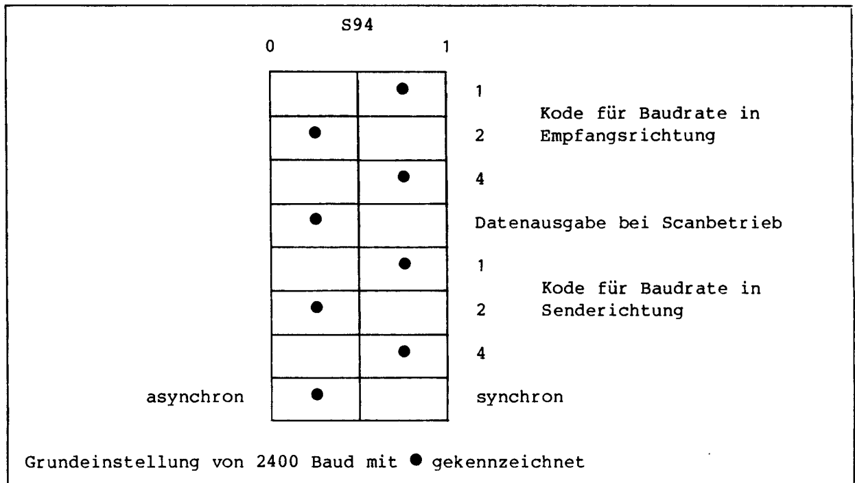
Bild 2.35 Funktionen des Schalters S94
