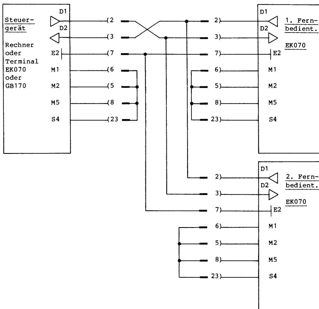
Bild 2.40 Zusammenschaltung mehrerer Geräte im QUASI-BUS-Betrieb
