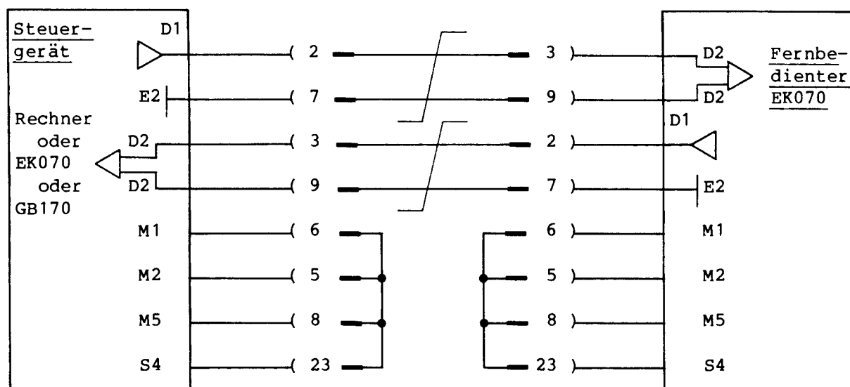
Bild 2.38 Zusammenschaltung von zwei Geräten nach V.10-Norm
