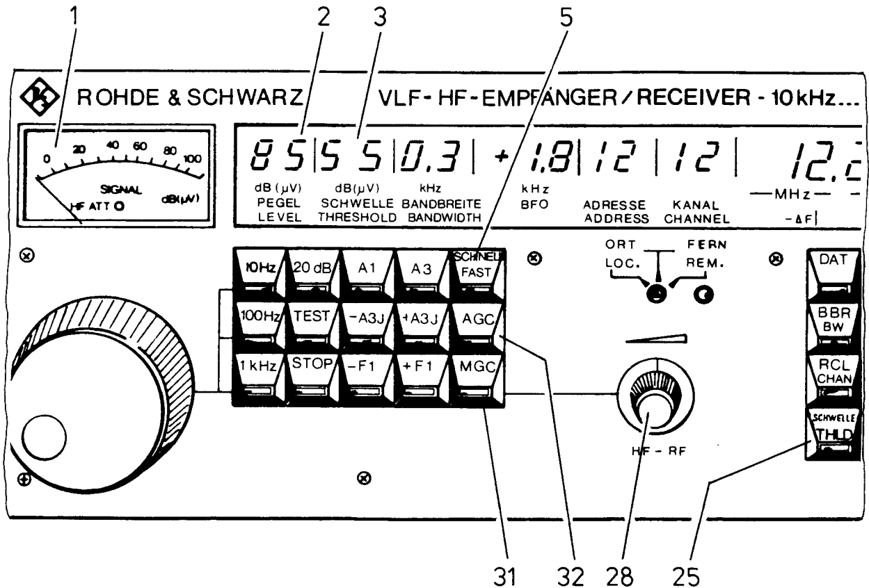
Bild 2.14 Anzeigen und Tasten für Regelarten- und Schwelleneinstellung
