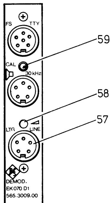
Bild 2.24 Leitungsausgänge
