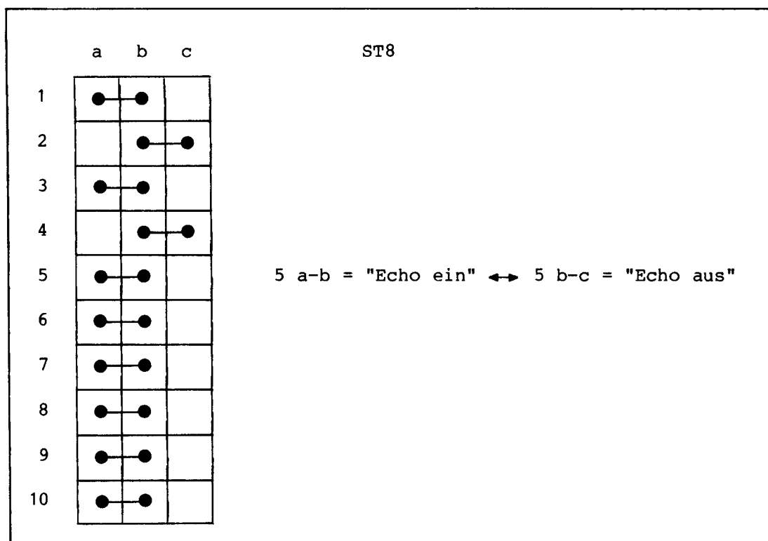
Bild 2.45 Kurzschlußstecker in Stellung "Echo ein"
