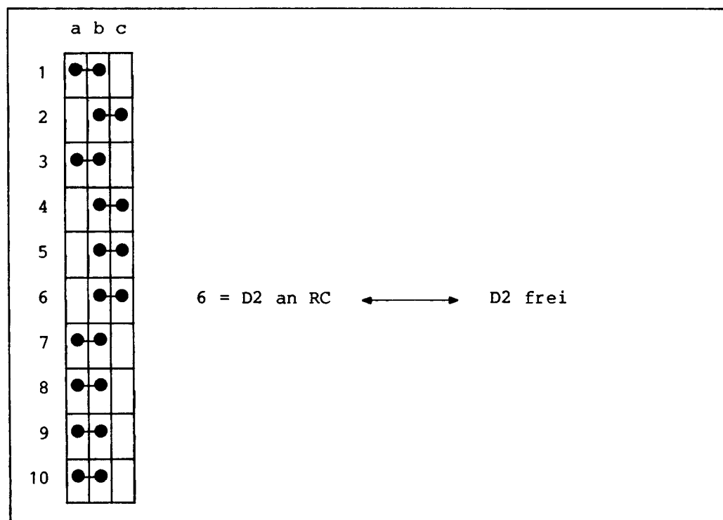
Bild 2.39 Kurzschluß-Stecker in Stellung V.10
