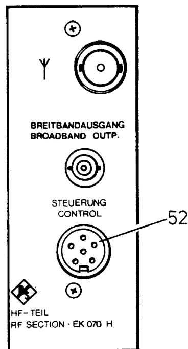
Bild 2.23 Steueranschluß
