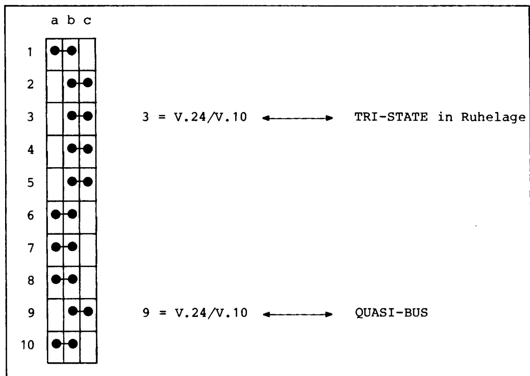
Bild 2.41 Kurzschluß-Stecker in Stellung QUASI-BUS
