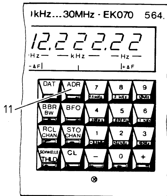
Bild 2.42 Adressenschalter
