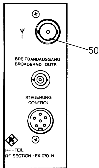
Bild 2.22 Antennenbuchse
