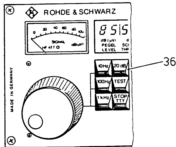
Bild 2.15 20dB-Taste
