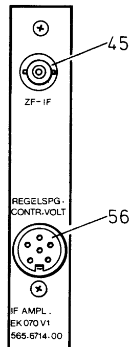
Regelspannungsausgang
