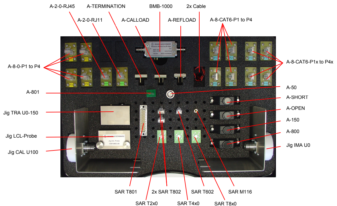
Bild 1 Bestandteile R&S ENY-FTS
