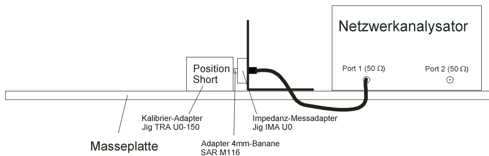
Bild 3 Kalibrieraufbau 'Kurzgeschlossen' für Asymmetrische Impedanz und Phasenwinkel
