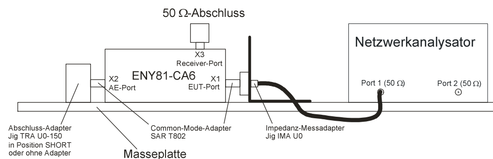
Bild 6 Messaufbau für Asymmetrische Impedanz und Phasenwinkel gemäß CISPR 16-1-2 für R&S ENY81-CA6
