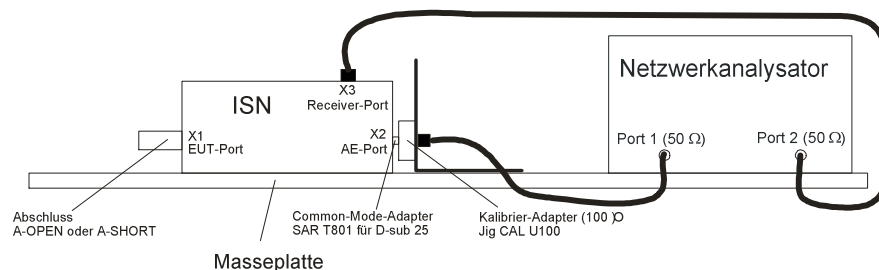
Bild 11 Messaufbau für Entkopplungsdämpfung gemäß CISPR 16-1-2
