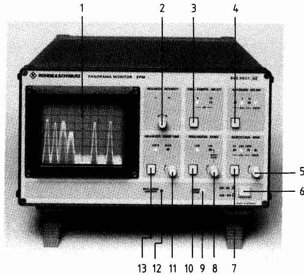
Bild 2-1 Frontansicht Fig. 2-1 Front view
