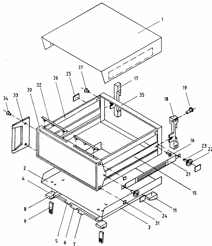
Frontrahmen- Frontseite
