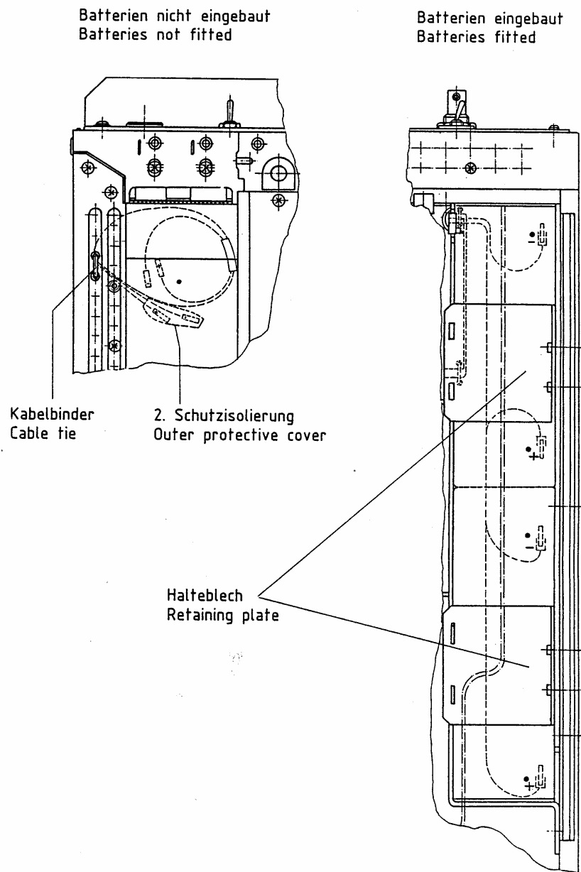
Bild 2-3 Einbau der Batterien Fig. 2-3 Fitting the batteries
