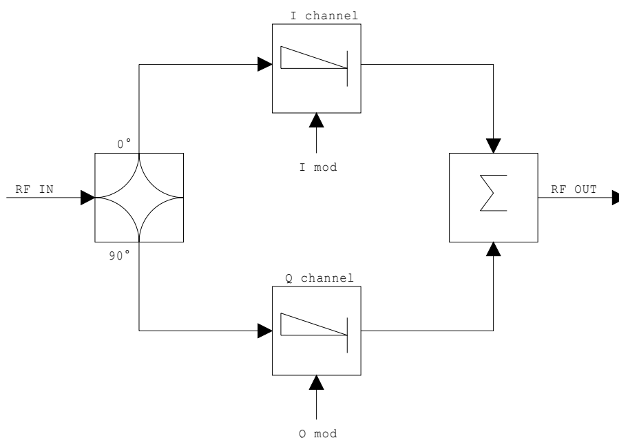
Fig. 4.27 I/Q modulation
