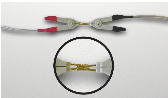
Abb. 3.1: Kurzschlussabgleich R&S®HZ184
