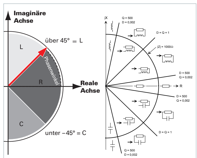
Abb.3.2: R&S®HM8118 Messprinzip schematisch links / detailliert rechts
