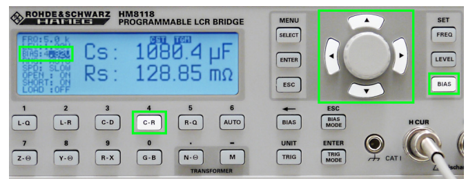
Abb. 7.3: Interne BIAS Vorspannung
