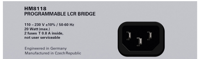
Abb. 4.1: Ansicht Kaltgeräteeinbaustecker
