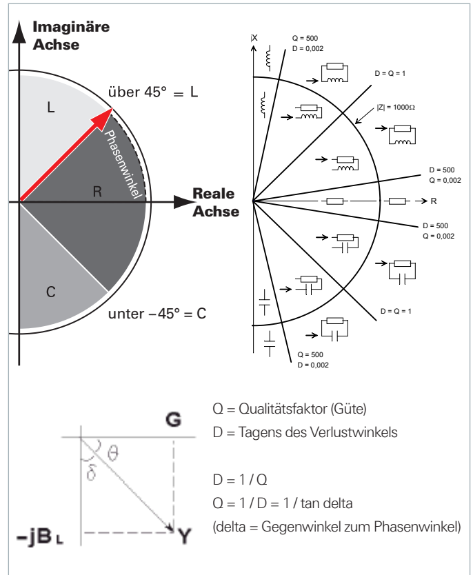
Abb. 4.3: Messprinzip
