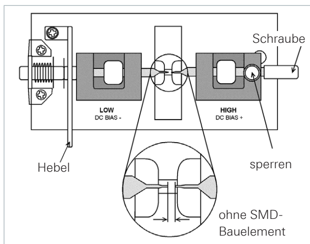
Abb. 8.13: Leerlaufabgleich mit R&amp;S®HZ188
