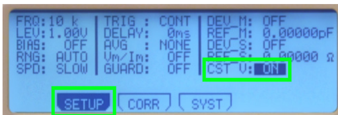
Abb. 7.2: Konstantspannung CST_V aktiviert
