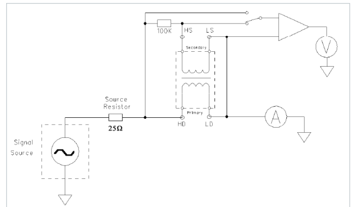
Abb. 8.9: Messung der Gegeninduktivität
