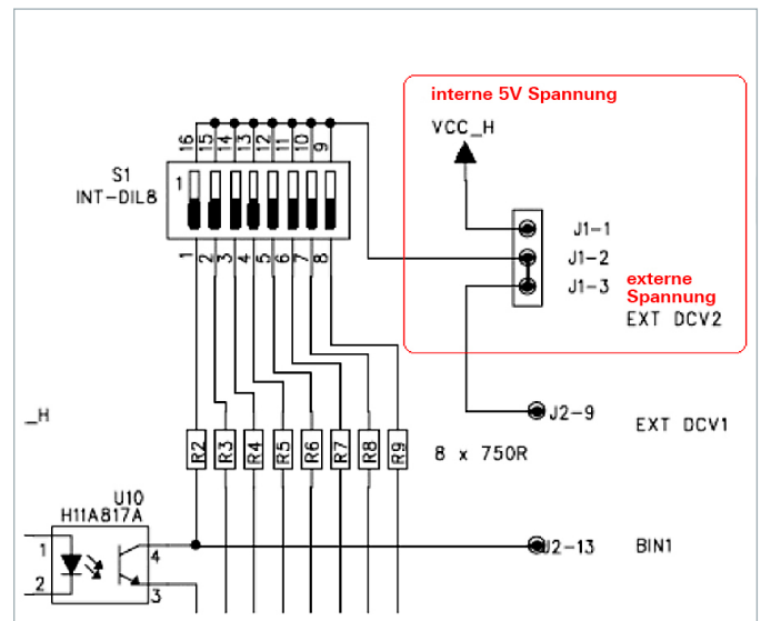
Abb. 8.16: R&S®HO118 interne Verschaltung
