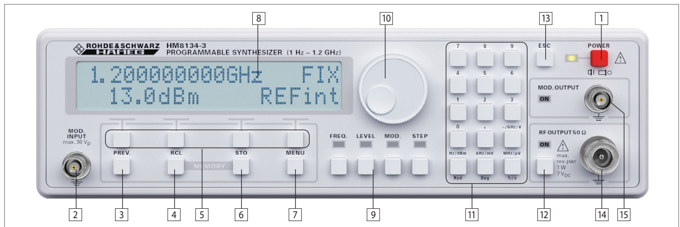
Abb. 2.1: Frontansicht des HM8134-3
