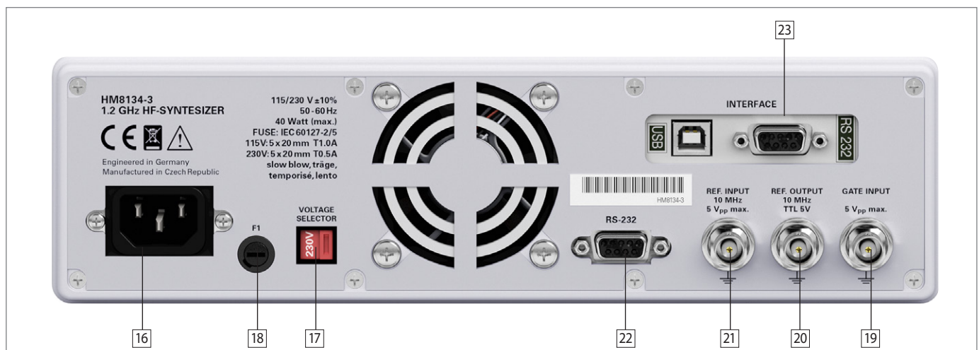
Abb. 2.2: Rückansicht des HM8134-3
