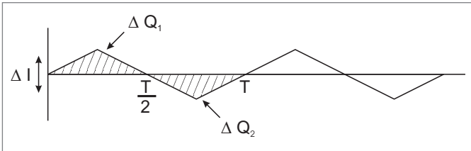
Abb. 3.4: Die Ladung eines Schaltnetzteiltes
