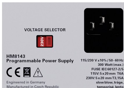
Abb. 1.1: Netzspannungswahlschalter HM8143
