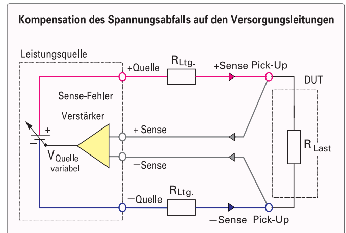
Abb. 4.1: Kompensation des Spannungsabfalls
