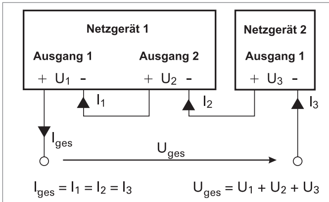
Abb. 3.5: Serienbetrieb
