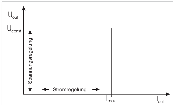
Abb. 3.7: Strombegrenzung
