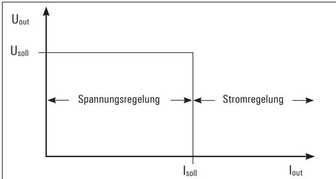
Abb. 4.5: Strombegrenzung
