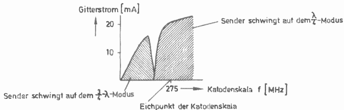
Bild 27 Abstimmverhalten des Senders bei Modulations - Betrieb (275...350 MHz)
