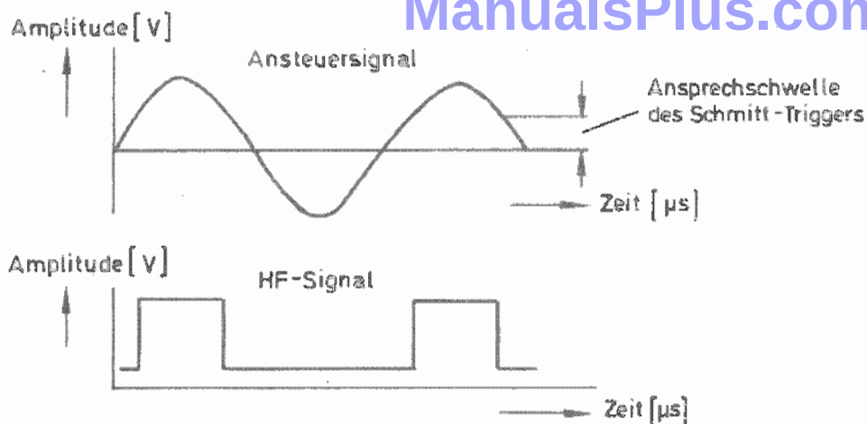
Bild 26 Ansteuerung des Senders in Stellung EXT. mit einem sinusförmigen Signal
