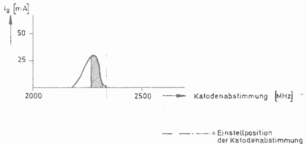
Bild 20 Prinzipieller Verlauf des Gitterstromes bei 500 MHz, 1200 MHz und 2300 MHz (abhängig von der Katodeneinstellung) bei 1000 V Anodenspg und entlastetem Sender
