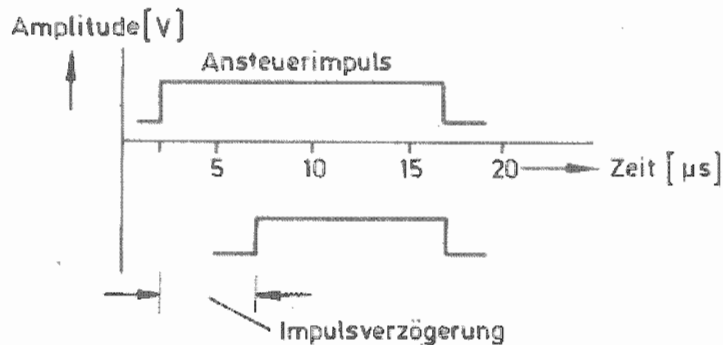
Bild 25 Korrektur der Anstiegsverzögerung des HF-Impulses durch einen längeren Ansteuerimpuls (geforderte Impulsdauer z.B. 10 \mu s)
