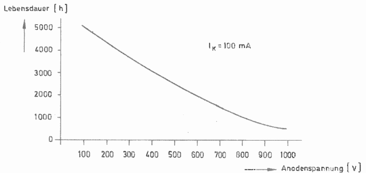
Bild 18 Mindestwert der zu erwartenden Lebensdauer der Oszillatordröhre in Abhängigkeit von der Anodenspannung
