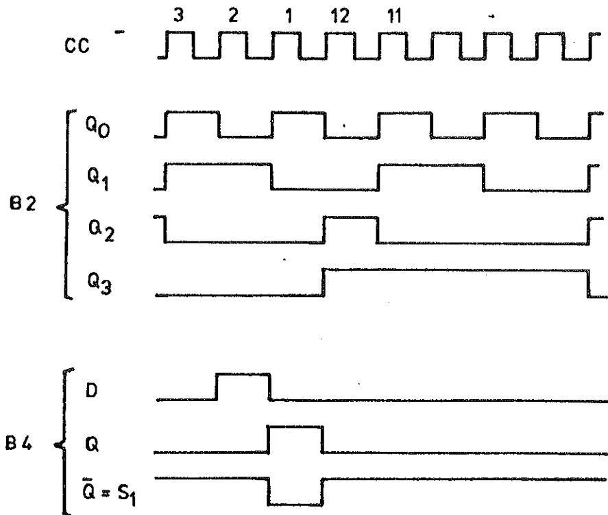
Bild 4-4 Pulsfolge der Zählerausgänge Q 0 ... Q 3
