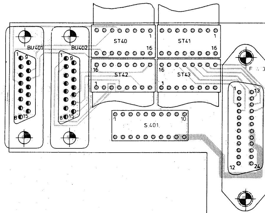
Ansicht und Leitungsführung Bauteilseite (Innenlage DV12) View of tracks on component side
