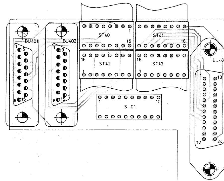
Ansicht und Leitungsführung Bauteilseite: (Innenlage DV41) View of tracks on component side
