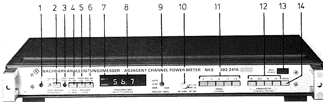
Bild 4 Frontansicht
