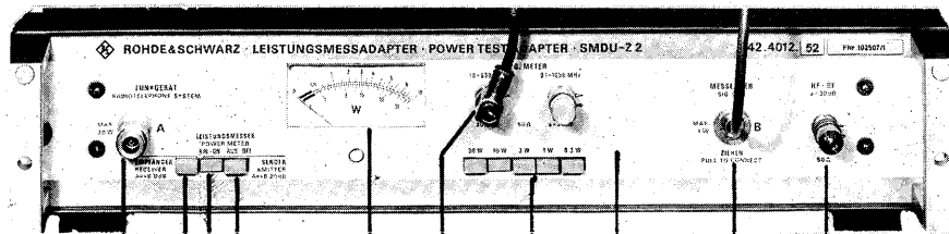
Leistungsmessadapter Power Test Adapter
