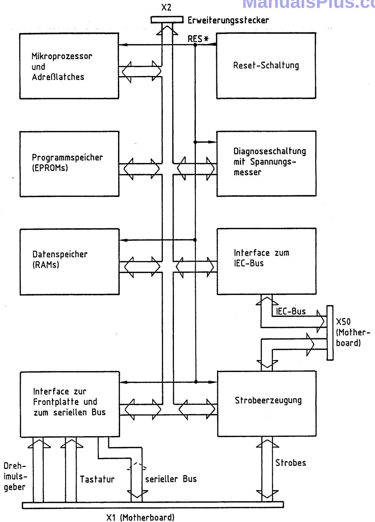
Bild 5-4 Blockschaltbild Rechner
