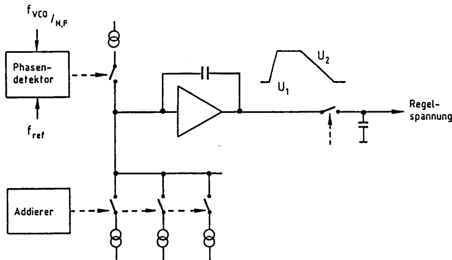
Bild 5-2 Blockschaltbild N,F-Regelschleife
