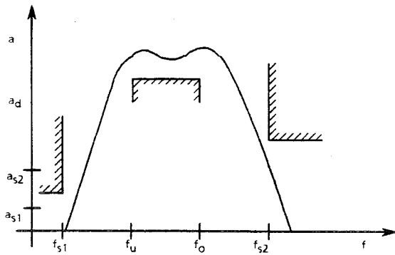
Bild 5-3 Filterdurchlaßkurve
