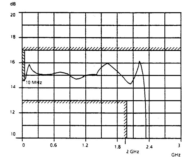
Bild 5-4 |S_{21}| typische Kurve und Toleranzfeld
