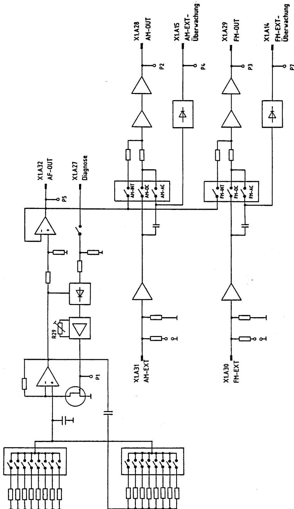
Bild 5-1 Blockschaltbild NF-Generator
