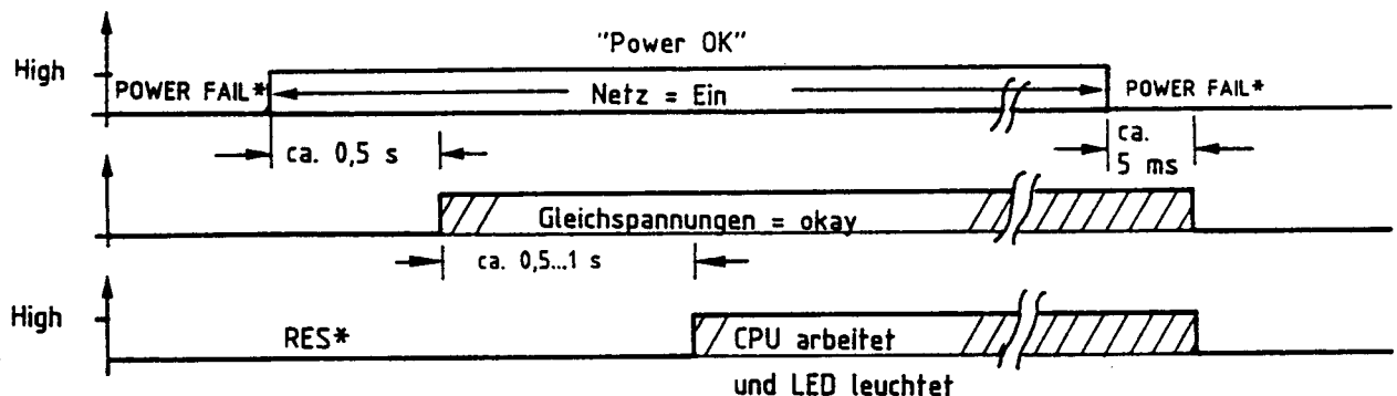
Bild 5-3 Netzteil Ein-/Ausschaltsequenzen (nicht maßstäblich)
