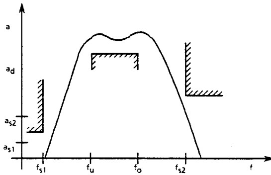
Bild 5-3 Filterdurchlaßkurve
