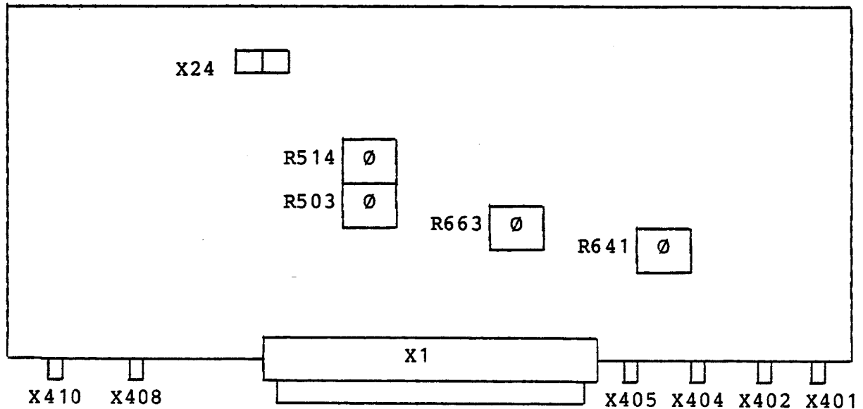
Bild 5-2 Anordnung der Ein-/Ausgänge und der Abgleichelemente
