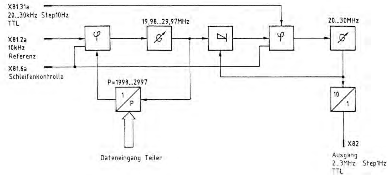
Bild 5-2 Blockschaltbild Interpolationsoszillator 1 kHz
