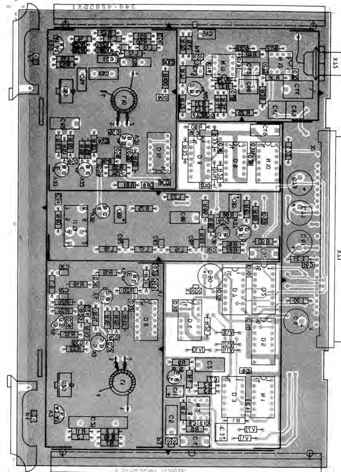
Ansicht und Leitungsführung Lotseite View of tracks on solder side
