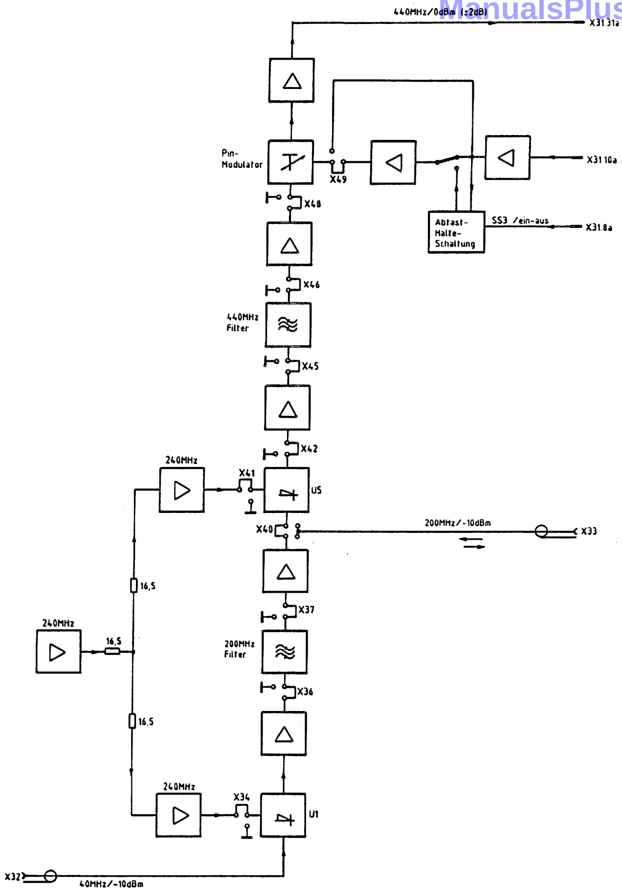
Bild 5-1 Blockschaltbild Mischer
