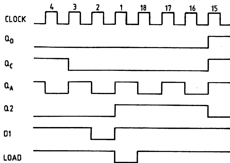
Bild 5-1 Pulsdiagramm des programmierbaren Teilers
