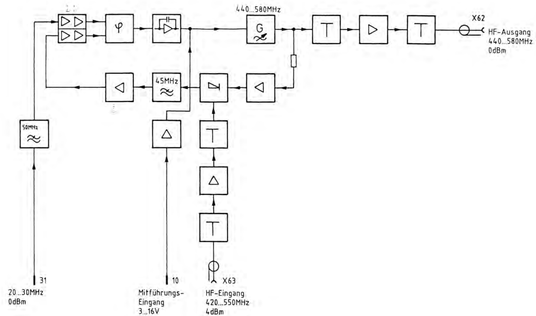
Bild 5-1 Blockschaltbild
