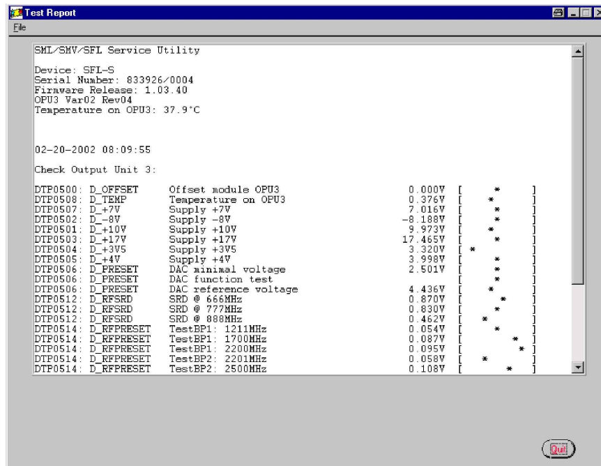
Bild 7.5-4: Test Report als Ergebnis des Modul Checks
