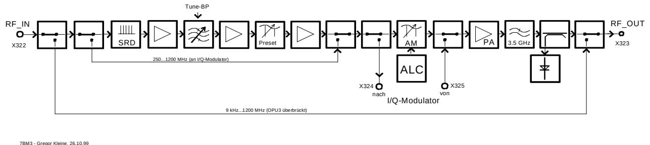
Bild 7.2 Vereinfachtes Blockschaltbild des Ausgangsteil 2 GHz / 3 GHz
