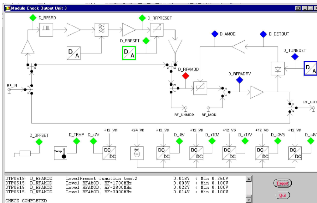
Bild 7.5-3 Blockschaftbild im Modul Check des Ausgangsteil 2 GHz / 3 GHz
