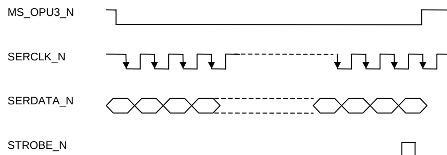
Bild 7.5.4 Impulsdigramm der digitalen Schnittstelle des OPU3
