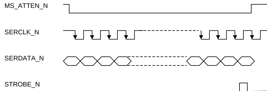
Bild 3-1 Eichleitungsprogrammierung, Zeitablauf an der Schnittstelle X301.
