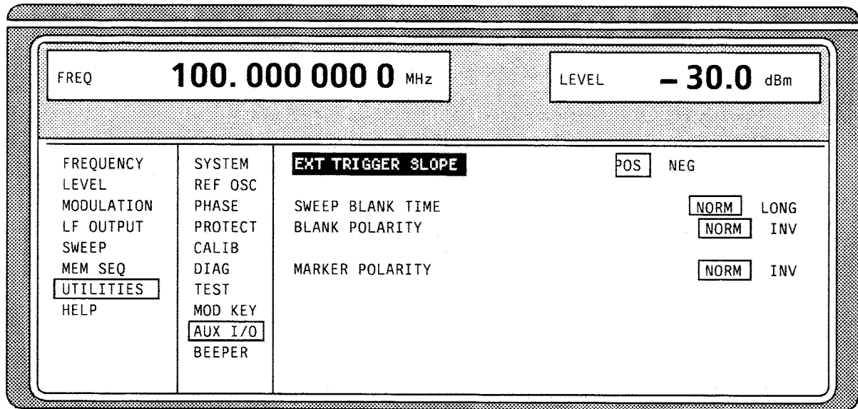
Bild 2-59 Menü UTILITIES - AUX I/O
