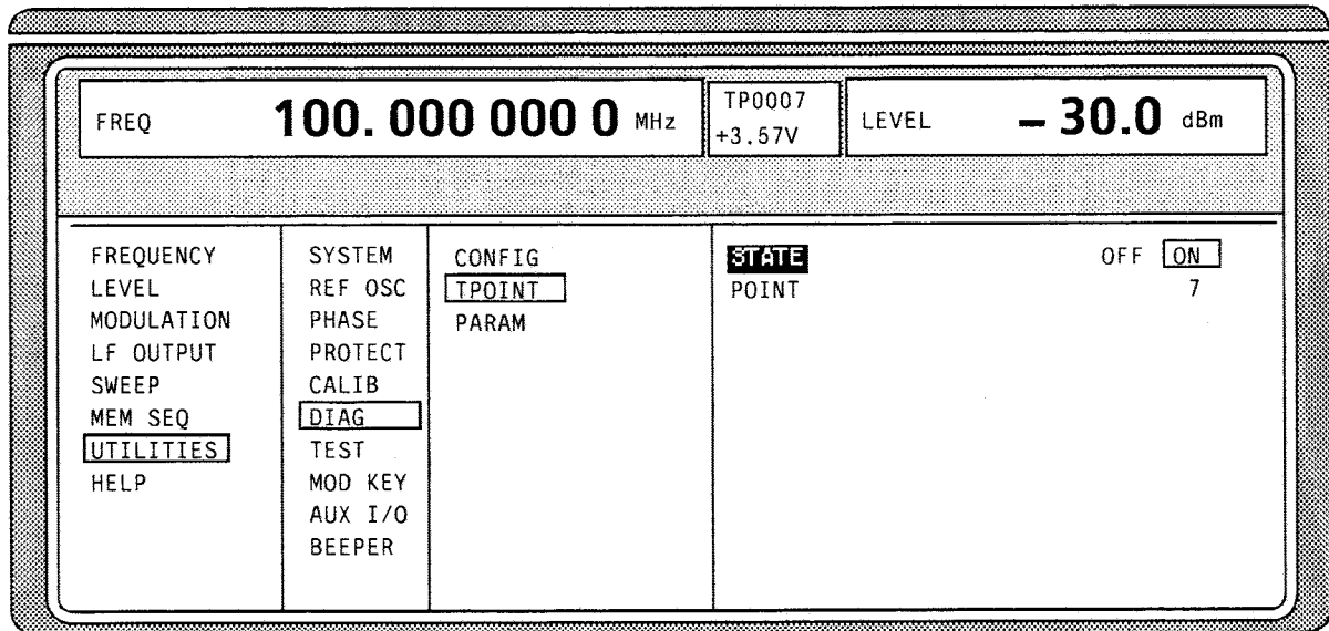
Bild 2-56 Menü UTILITIES-DIAG-TPOINT
