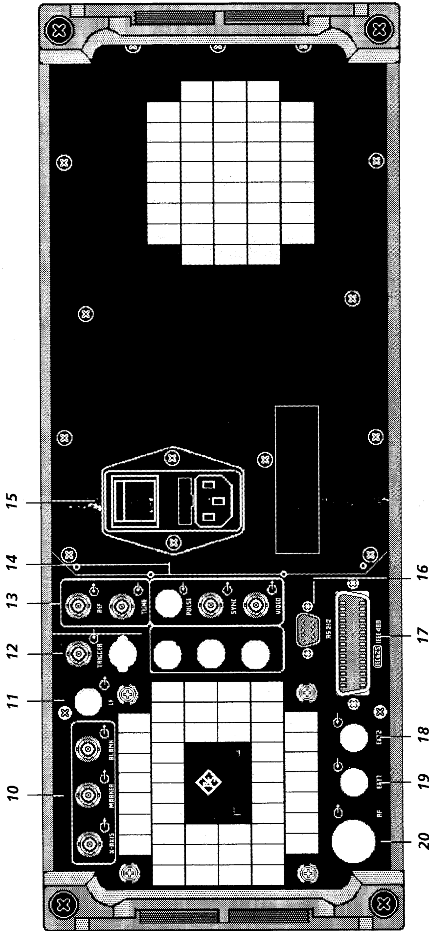
Bild 2-2 Rückansicht
