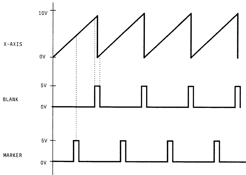
Bild 2-38 Signalbeispiel Sweep: MODE = AUTO, BLANK TIME = NORMAL
