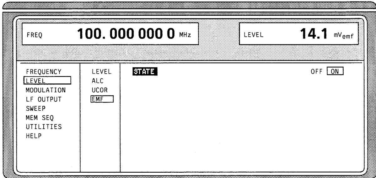
Bild 2-23 Menü LEVEL-EMF
