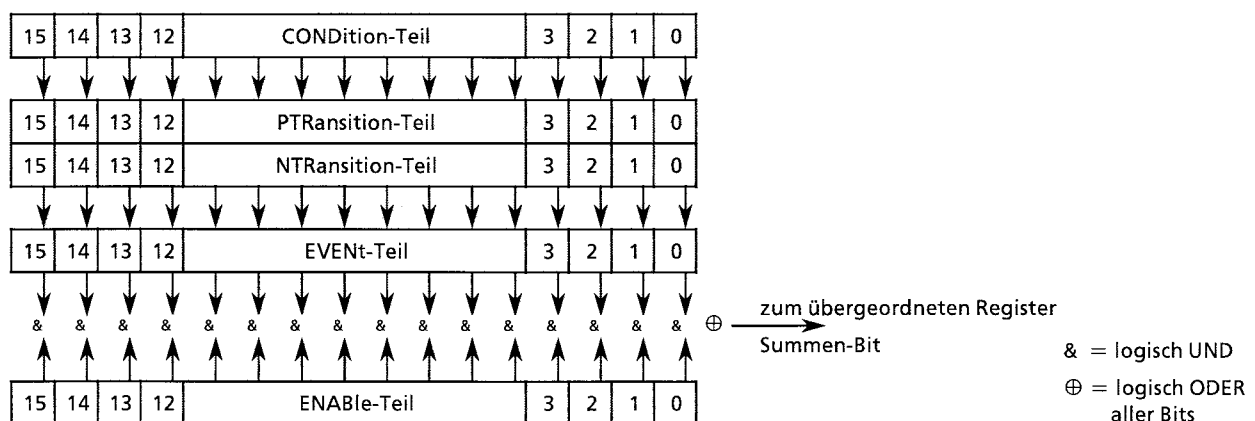
Bild 3-3 Das Status-Register-Modell
