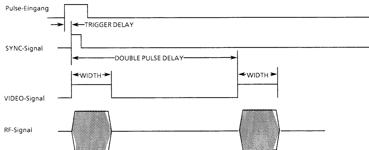
Bild 2-30 Signalbeispiel 2: Doppelpuls, TRIGGER MODE = EXT, SLOPE = POS
