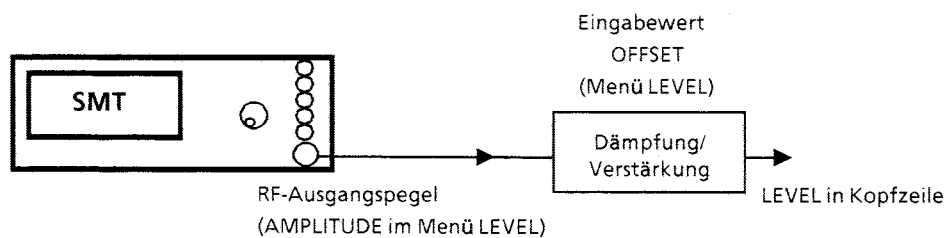
Bild 2-19 Beispiel für eine Schaltung mit Pegeloffset
