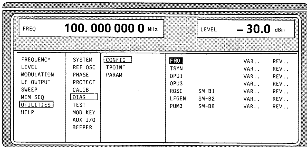
Bild 2-55 Menü UTILITIES-DIAG-CONFIG
