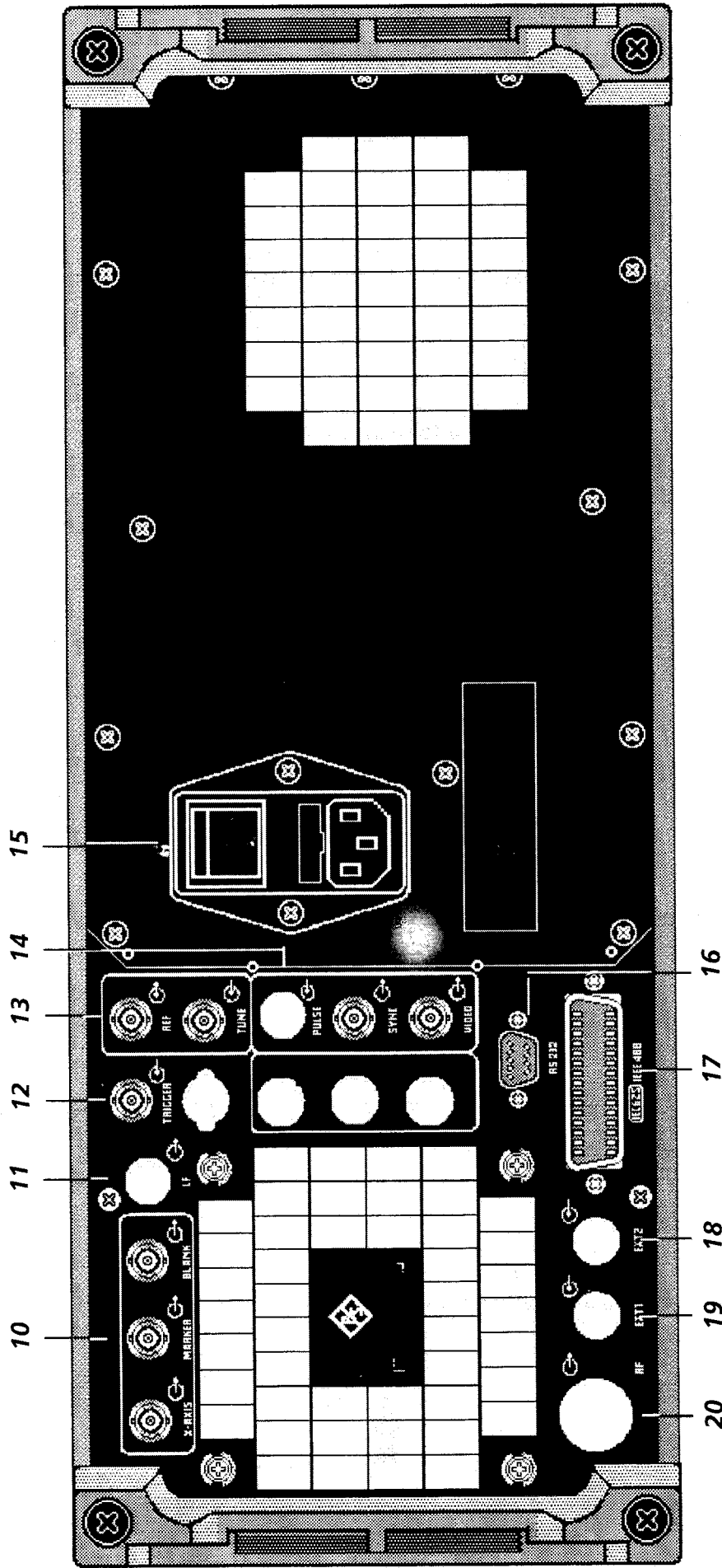
Bild 2-2 Rückansicht
