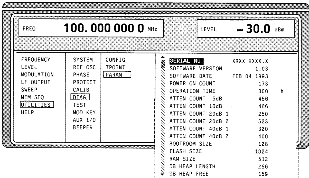
Bild 2-57 Menü UTILITIES-DIAG-PARAM
