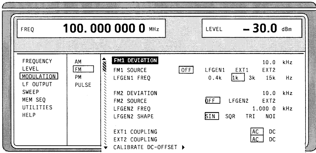
Bild 2-25 Menü MODULATION-FM (Preseteinstellung), Ausstattung mit Option SM-B2, LF-Generator (LFGEN2).
