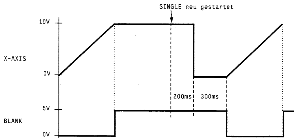
Bild 2-39 Signalbeispiel Sweep: MODE = SINGLE, BLANK TIME = LONG
