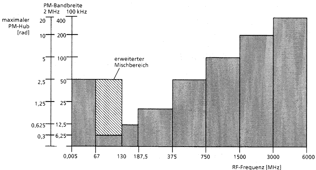
Bild 2-28 Abhängigkeit des PM-Maximalhubs von der eingestellten RF-Frequenz
