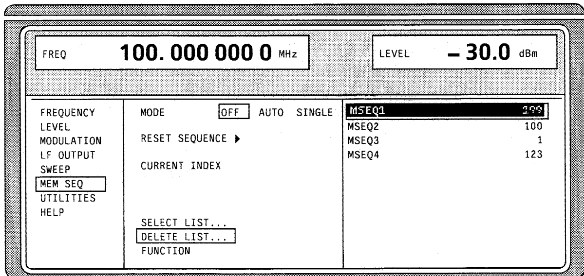
Bild 2-9 DELETE-LIST-Auswahlfenster
