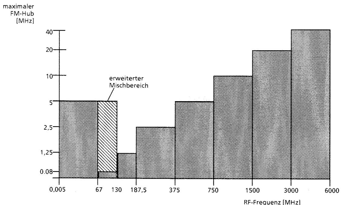
Bild 2-26 Abhängigkeit des FM-Maximalhubs von der eingestellten RF-Frequenz
