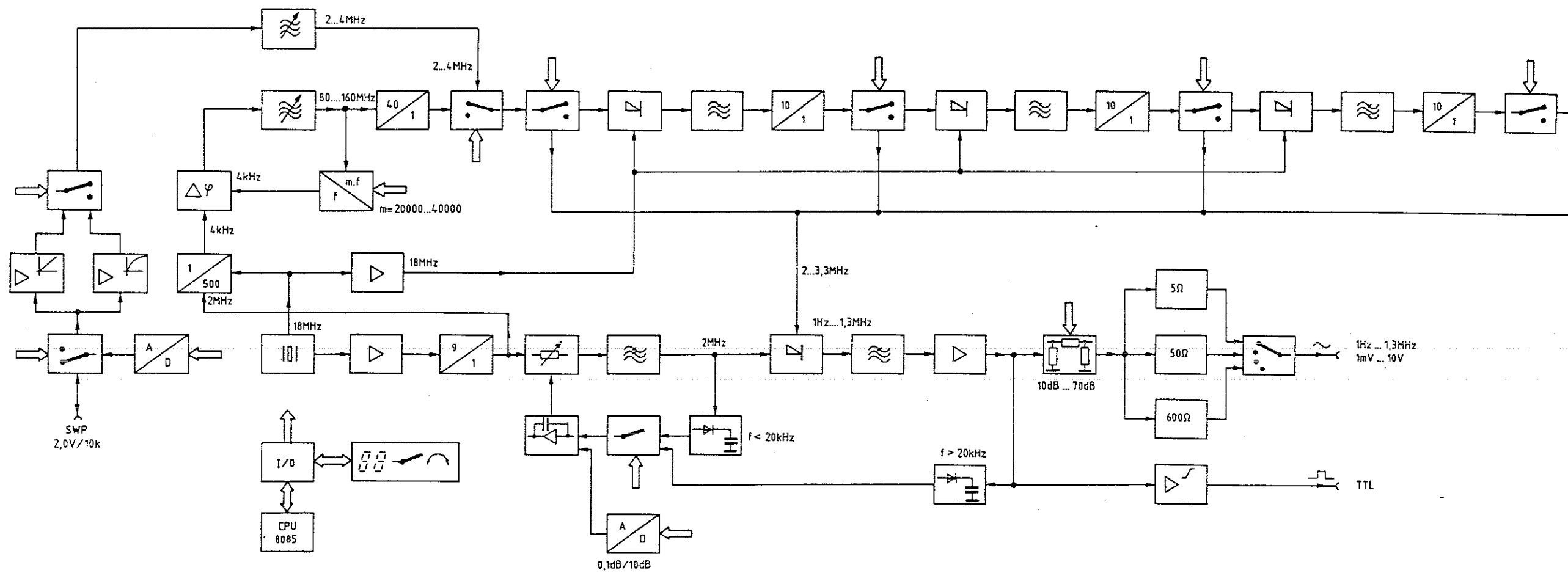
Bild 4-1 Blockschaftbild des Generators SPN Fig. 4-1 Block diagram of the Generator SPN
