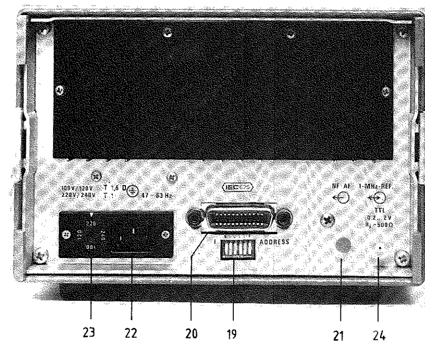
Bild 2-8 Rückansicht Fig. 2-8 Rear panel
