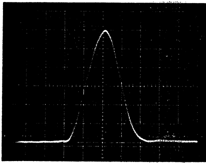
BILD 4 Links: 2T-Impuls, gemessen mit dem Kontrolloszillografen OKF. Zeitmaßstab 100 ns/cm, Belichtungszeit 1 s, Blende 8, Abbildungsmaßstab 1:1,2, Verschuß manuell ausgelöst.
