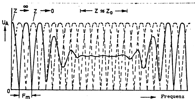
Bild 2-3 Frequenzabhängige Welligkeit
