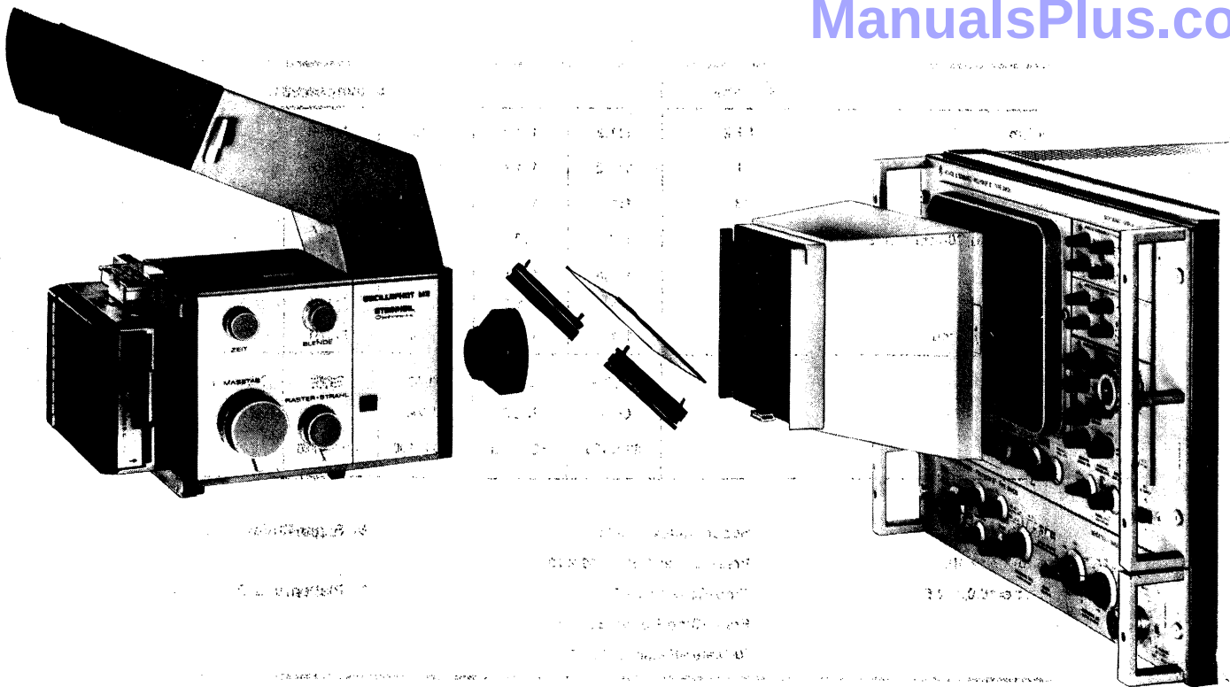
BILD 2 Oscillophot M2 mit Linse, Lichtteiler, Lichtteiler-Adapter und Anschlußflansch für Schirmbildaufnahmen am Polyskop III SWOB.
