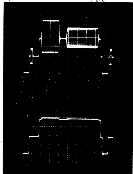
BILD 3 Zweifelaufnahme vom OKF-Bildschirm im Maßstab 1:2. Periodischer Vorgang 1/5 s, Blende 5,6. Oben: Prüfzelle 331; unten: die gleiche Prüfzelle nach Durchlaufen des OKF-Tiefpasses ( f_g = 1 MHz, Farbträger unterdrückung 45 dB) zur Auswertung der Intermodulation.
