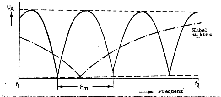
Bild 2-2 Spannungsverlauf am Bildschirm
