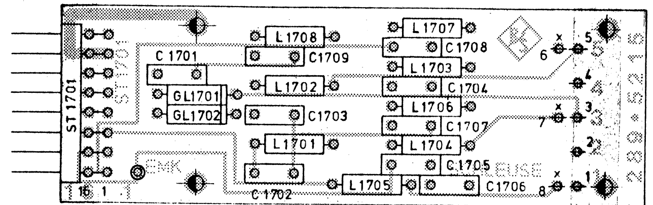
Ansicht und Leitungsführung Bauteilseite; View of components side with tracks
