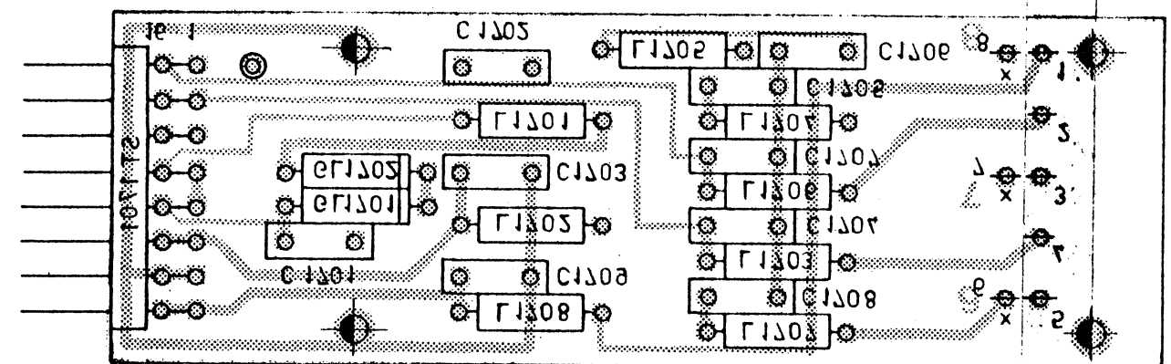
Ansicht und Leitungsführung Leiterseite View of printed side with tracks
