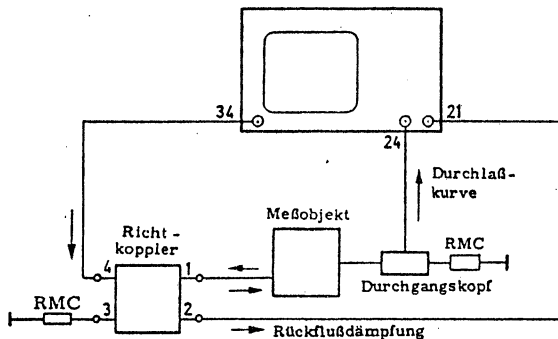
Bild 2-4 Messung der Rückflußdämpfung
