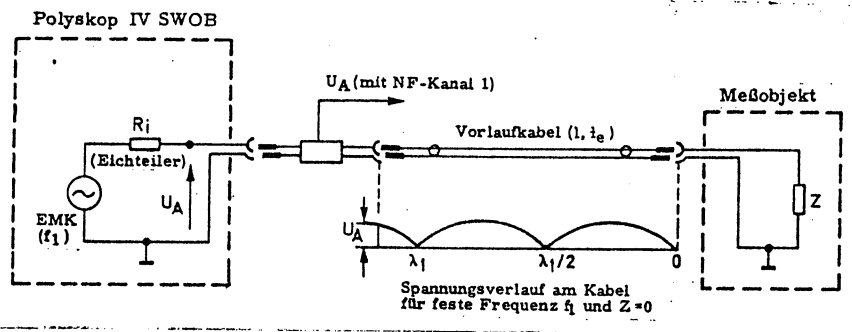
Bild 2-1 Reflexionsmessung mit Vorlaufkabel
