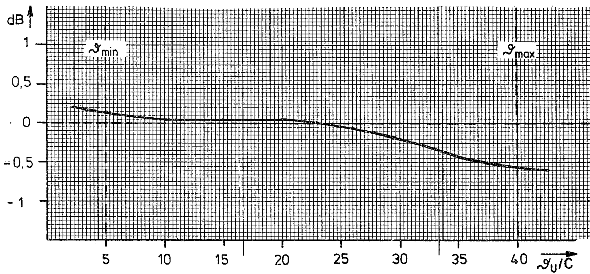
Bild 1-2 Typischer Temperaturgang
