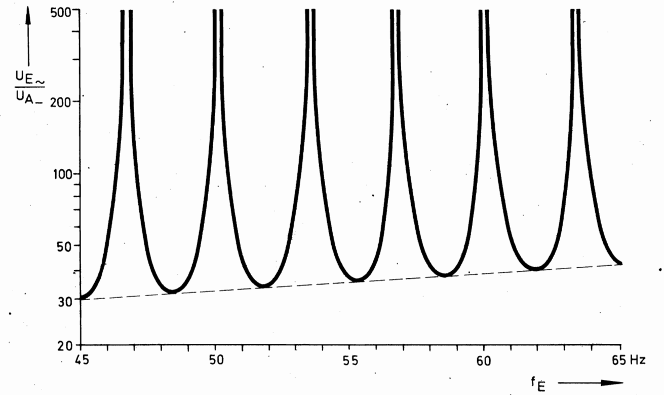
Bild 2-4 Störspannungsunterdrückung ManualsPlus.com
