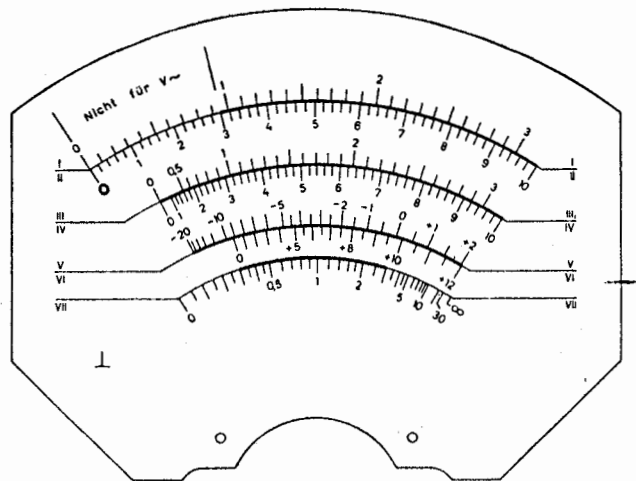
Bild 2. Skala des Anzeigeinstrumentes
