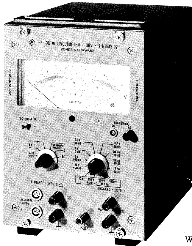
RF DC Millivoltmeter URV 216.3612.02
