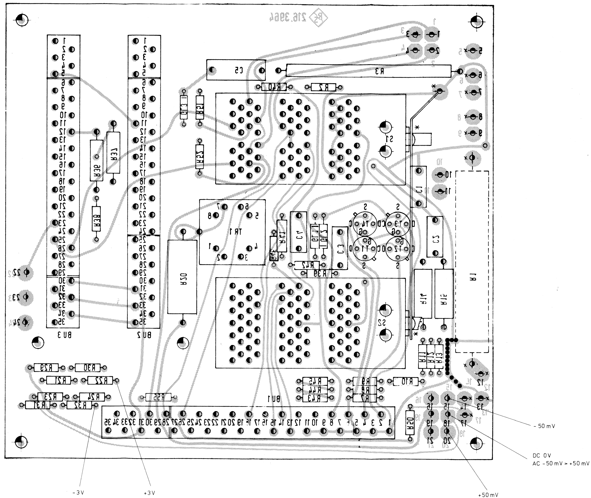
Ansicht und Leitungsführung Leiterseite
