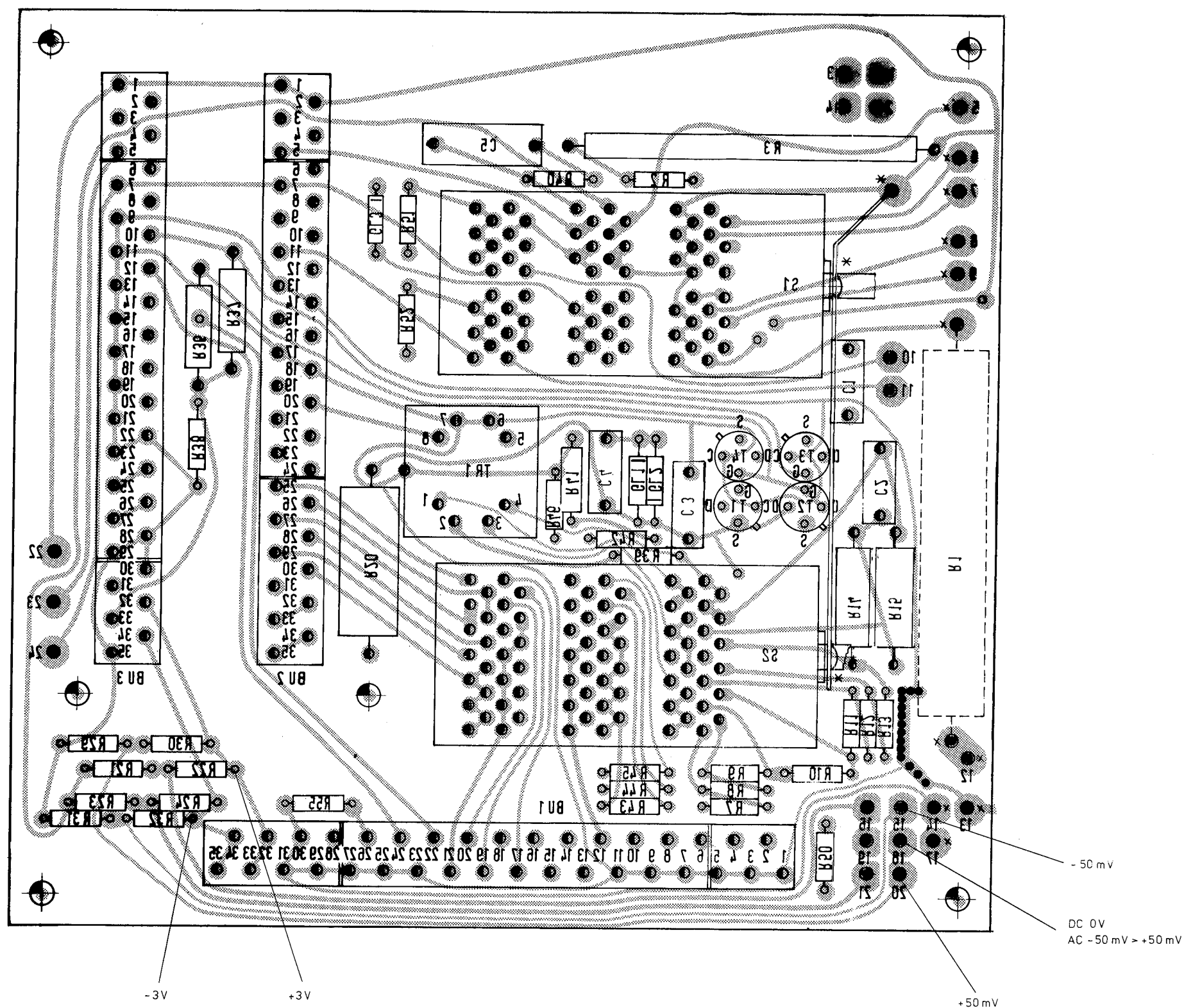
Ansicht und Leitungsführung Leiterseite
