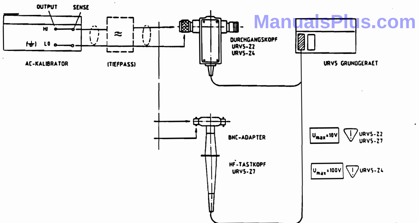
Bild 3-2 Überprüfung der AC-Meßgenauigkeit
