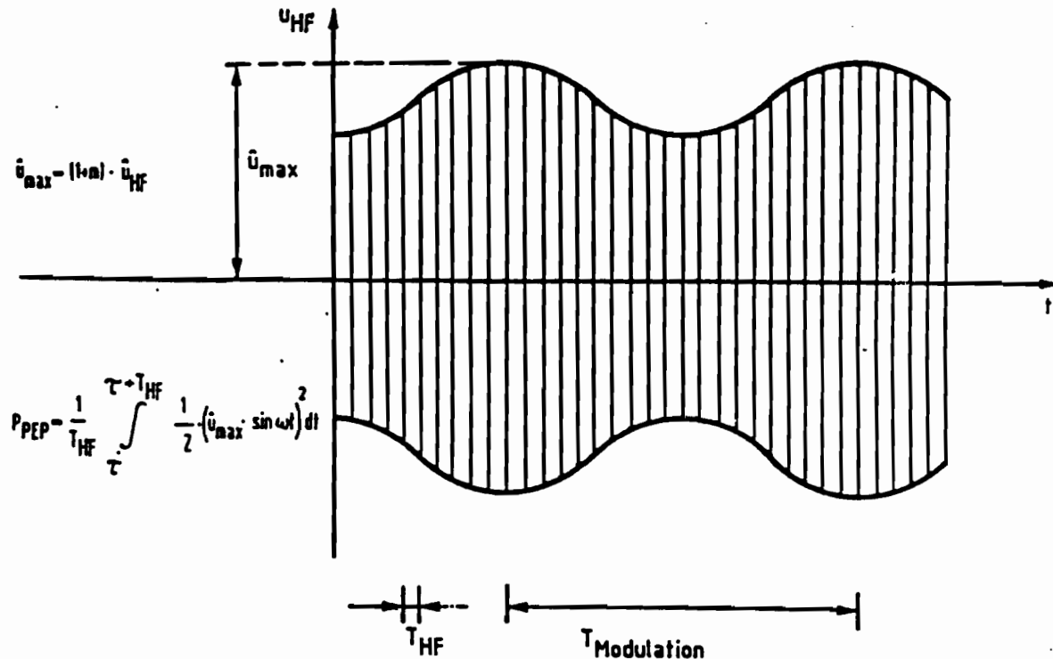
Bild 2-8 AM-modulierte HF-Spannung
