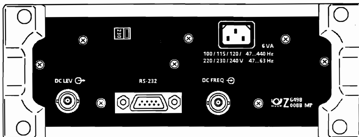
Bild 3-3 Rückansicht Variante 03
