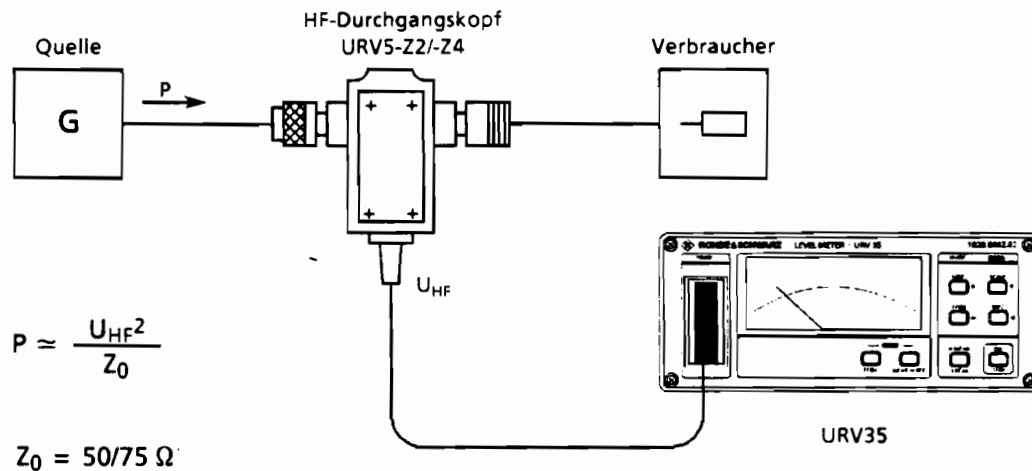
Bild 2-6 HF-Pegelmessung mit Durchgangsmeßkopf und URV35
