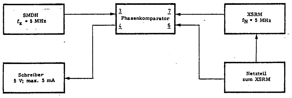
Bild 4 Meßaufbau zum Kalibrieren des Dekadischen HF-Meßsenders SMDH
