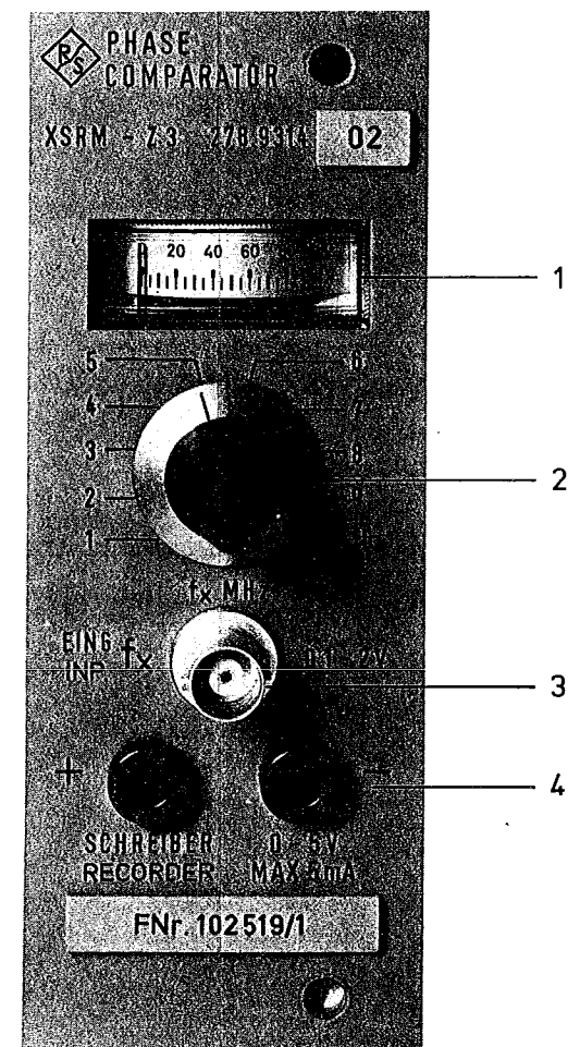
Bild 7 Frontansicht
