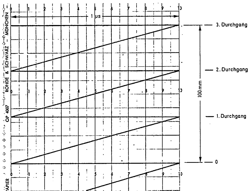
Bild 2 Registrierung mehrerer Phasendurchgänge (Vorschub 10 mm/min)
