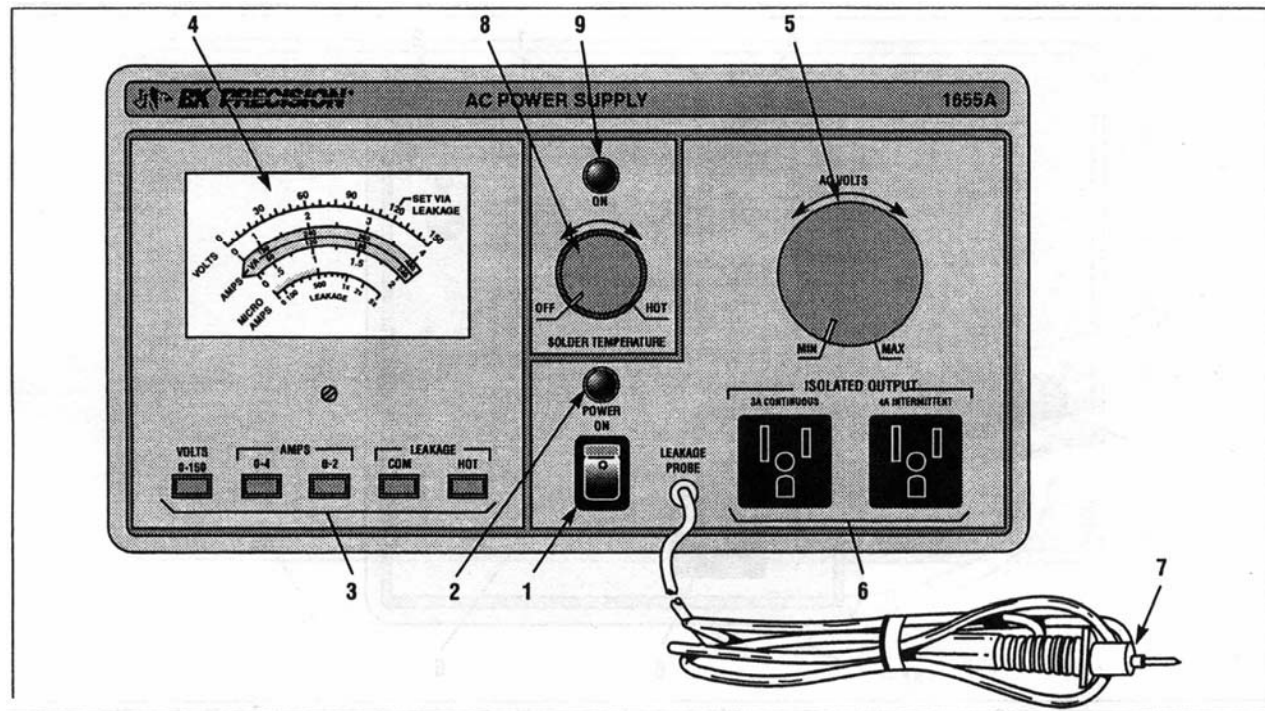
Figura 1. Controles e indicadores frontales del modelo 1655A
