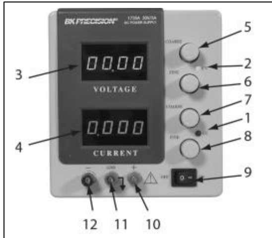
Figura 1. Controles e indicadores de el panel delantero
