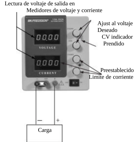
Figura 4. Típica operación de voltaje constante
