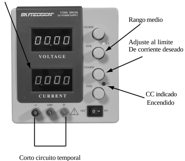
Figura 5. Estableciendo el limite de corriente
