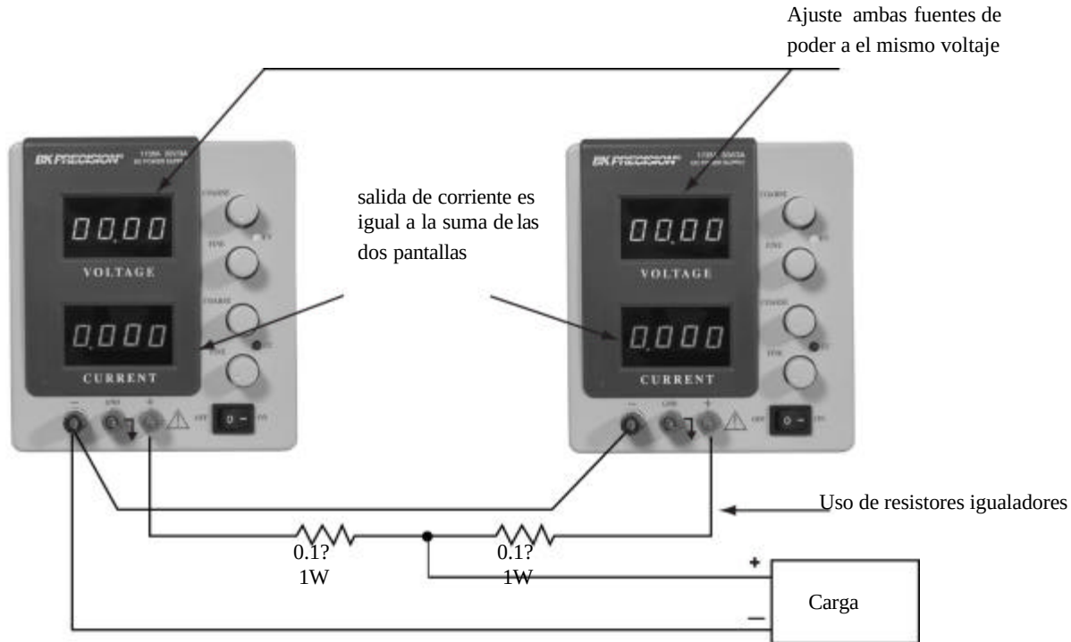
Figura 9. Conectando dos fuentes de poder en paralelo
