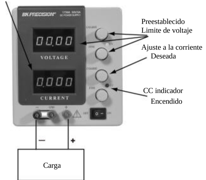
Figura 6. Tipica operación de corriente
