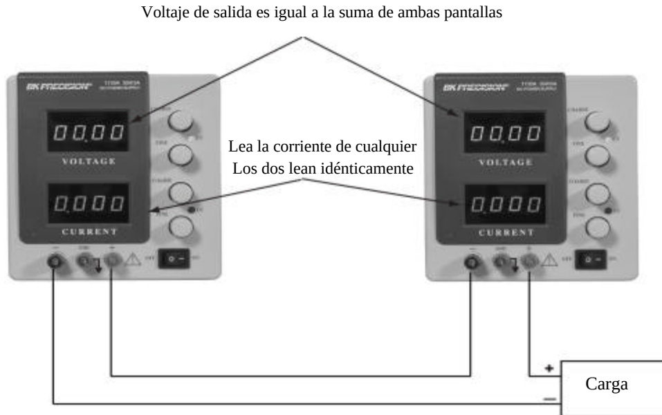
Figura 8 .Conectando dos fuentes de poder en serie
