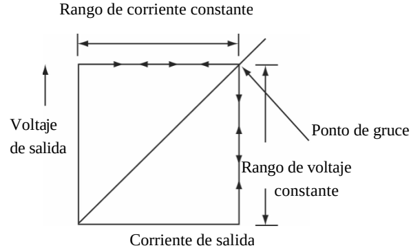
Figura 7. Voltaie constante/Corriente constante características
