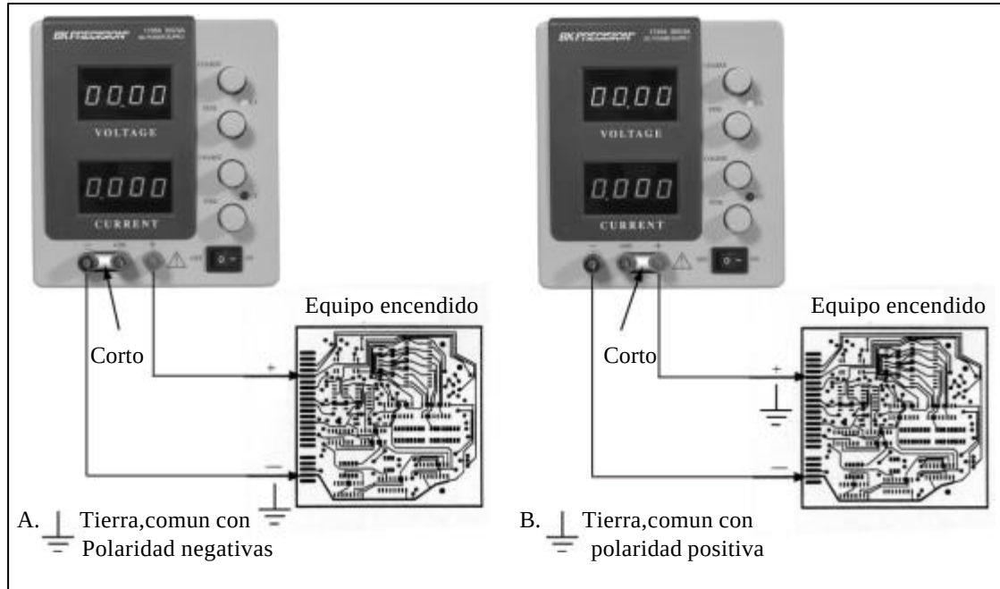
Figura A y B .Posibilidades de conecciones etierra
