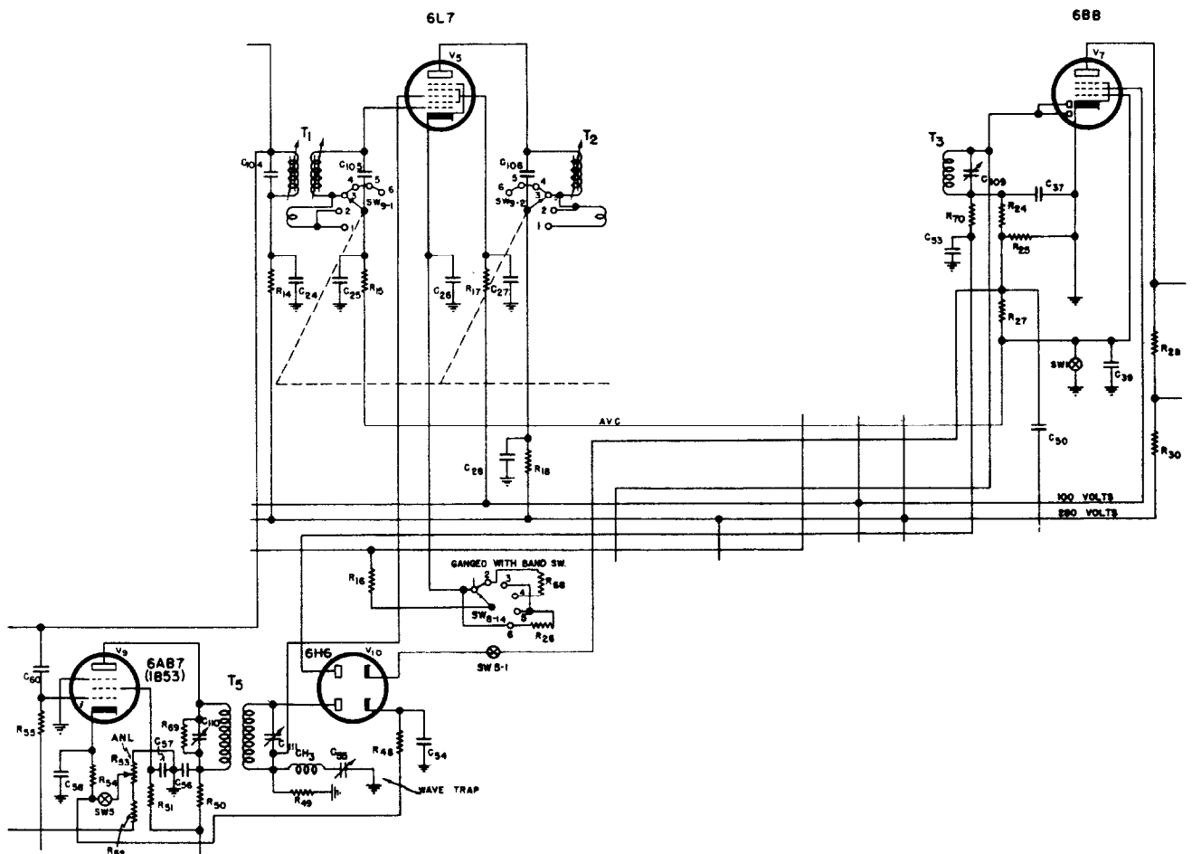
FIG. 5—NOISE LIMITER SCHEMATIC
