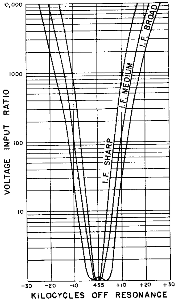
FIG. 1—I. F. SELECTIVITY
