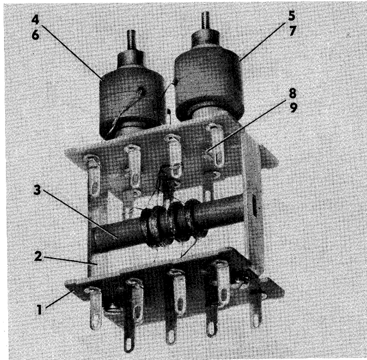
Figure 39. I-F Subassembly
