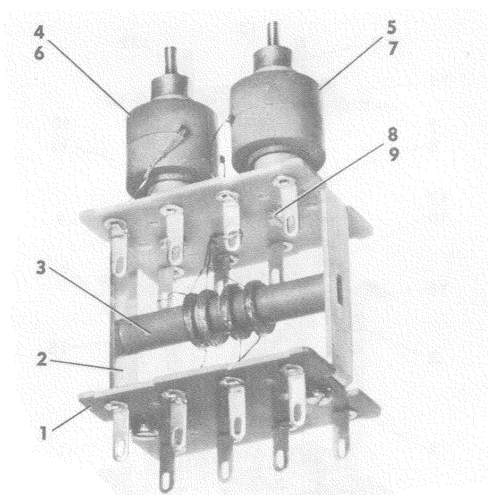
Figure 39. I-F Subassembly
