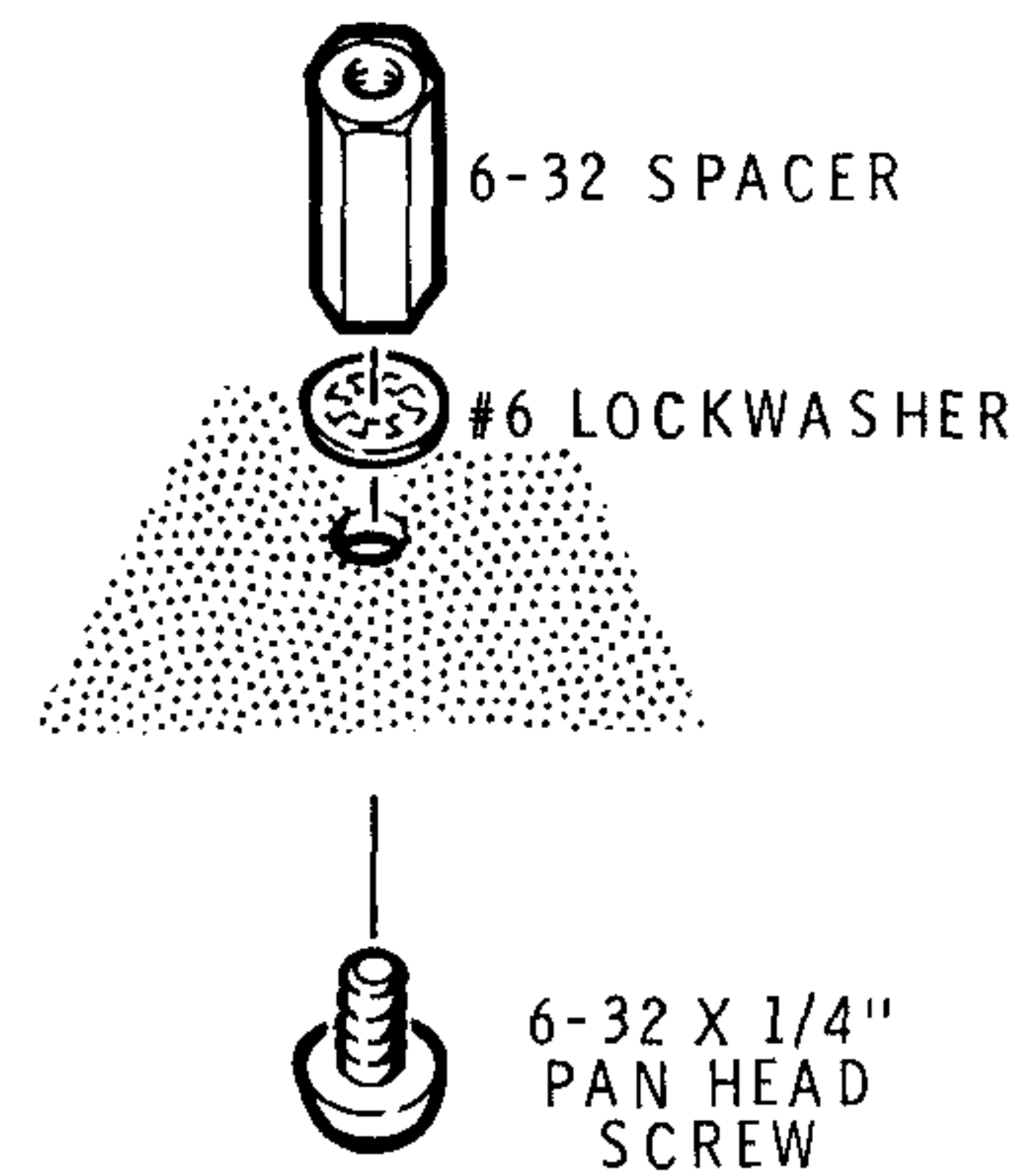
Detail 2-7E
