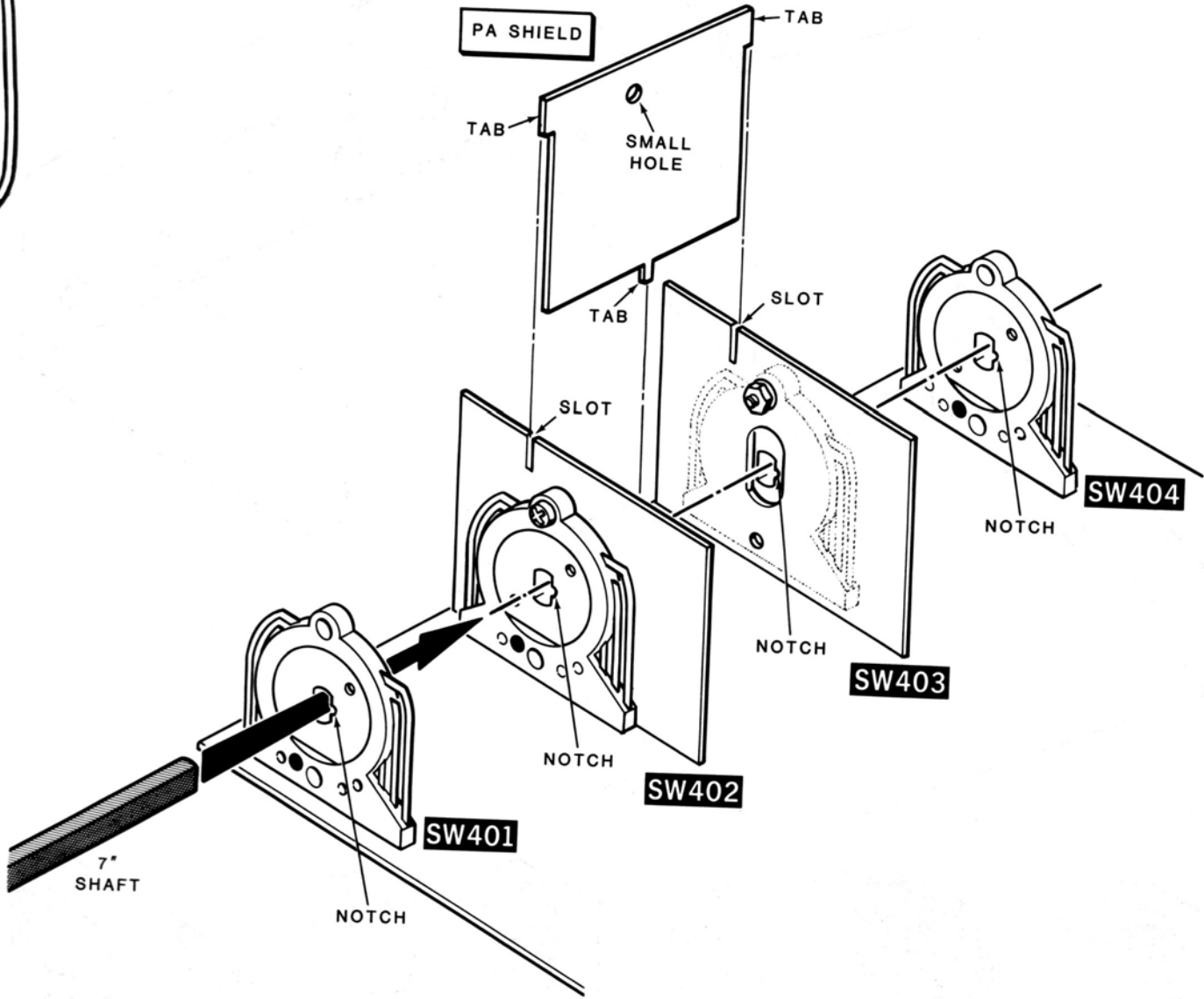
Detail 2-9E
