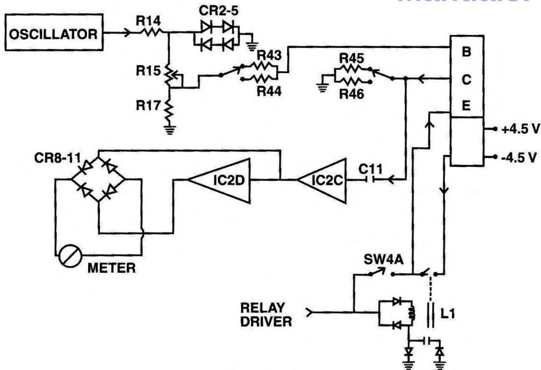
Fig. 20: Beta Test Circuit.
